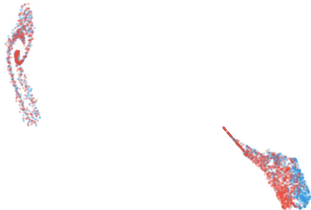
UMAP
