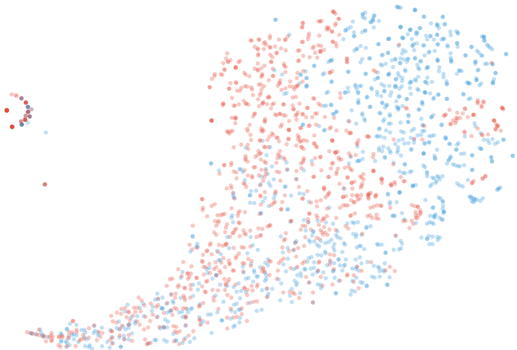
t-SNE
