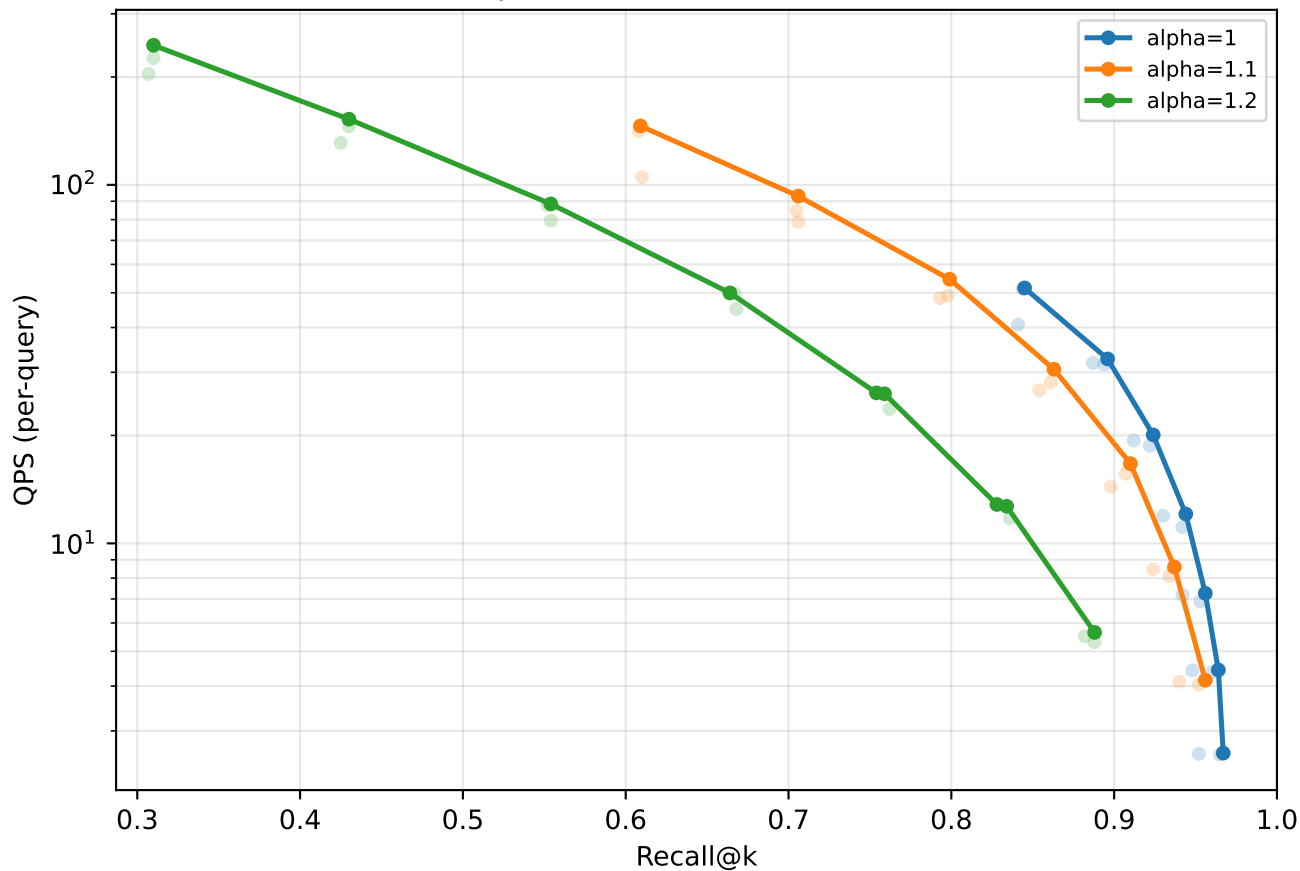
fiqa: Vamana ablation Pareto
