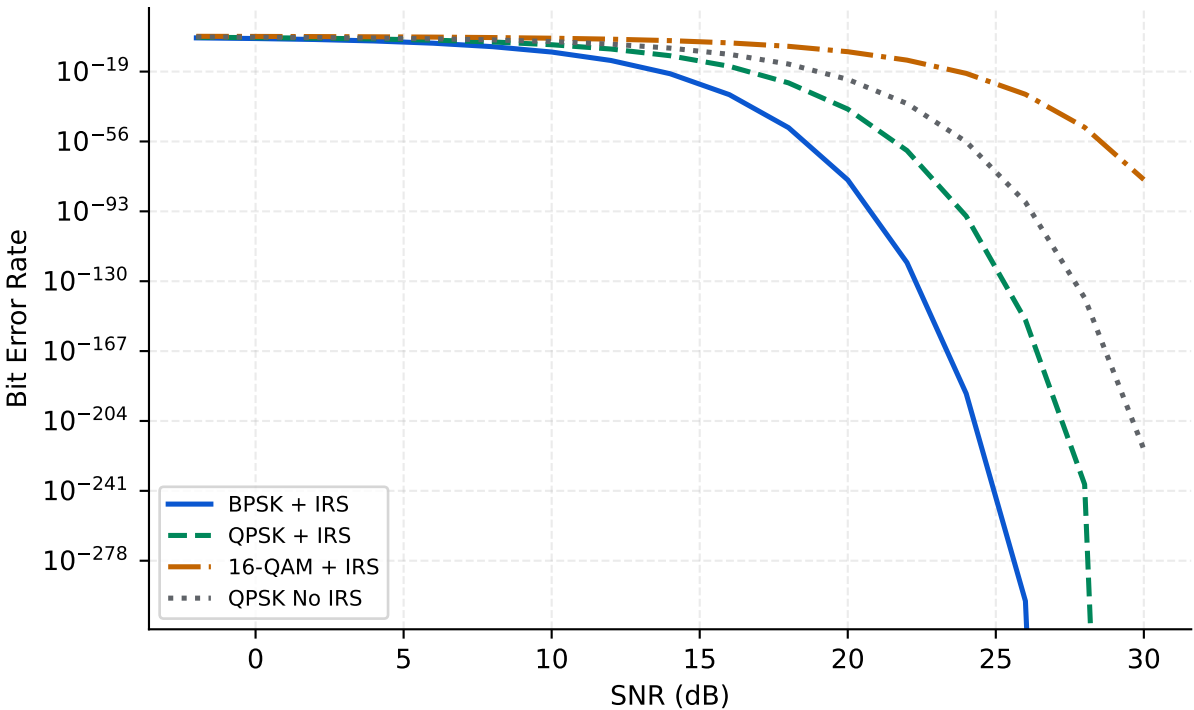
BER versus SNR
