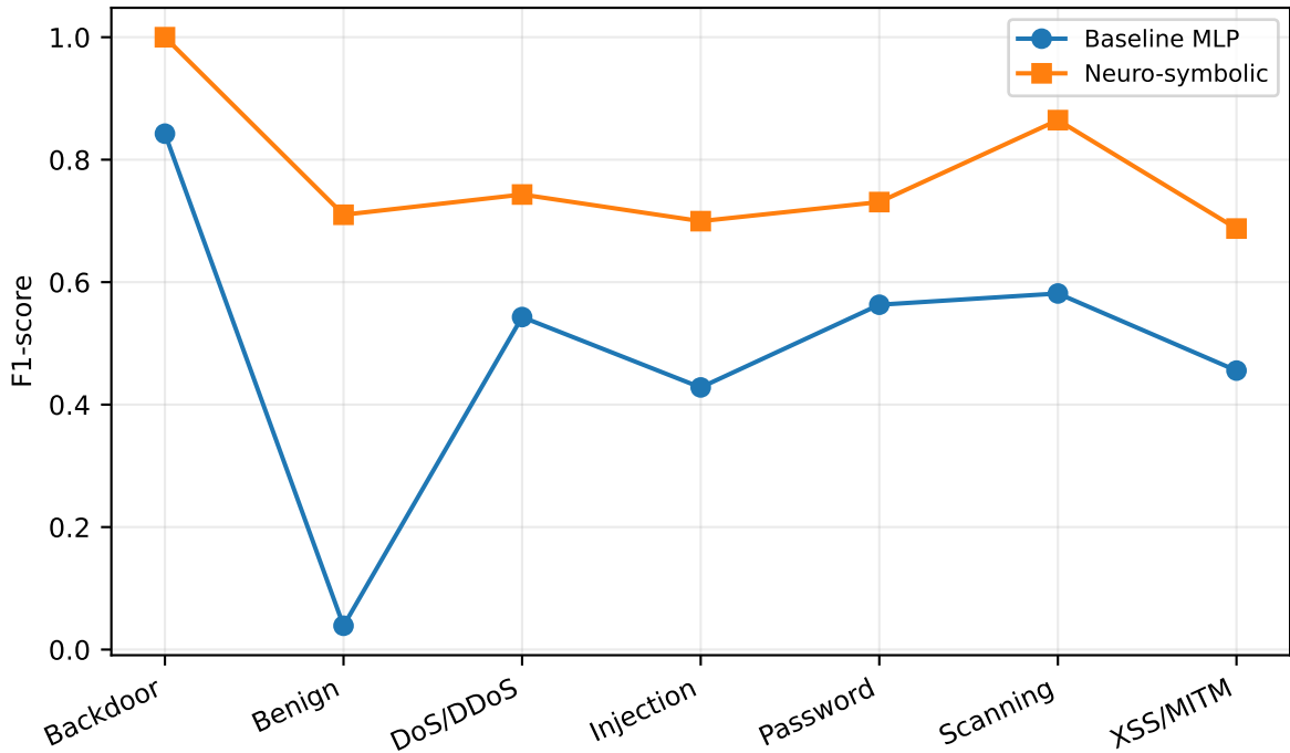
Per-Class F1 Comparison
