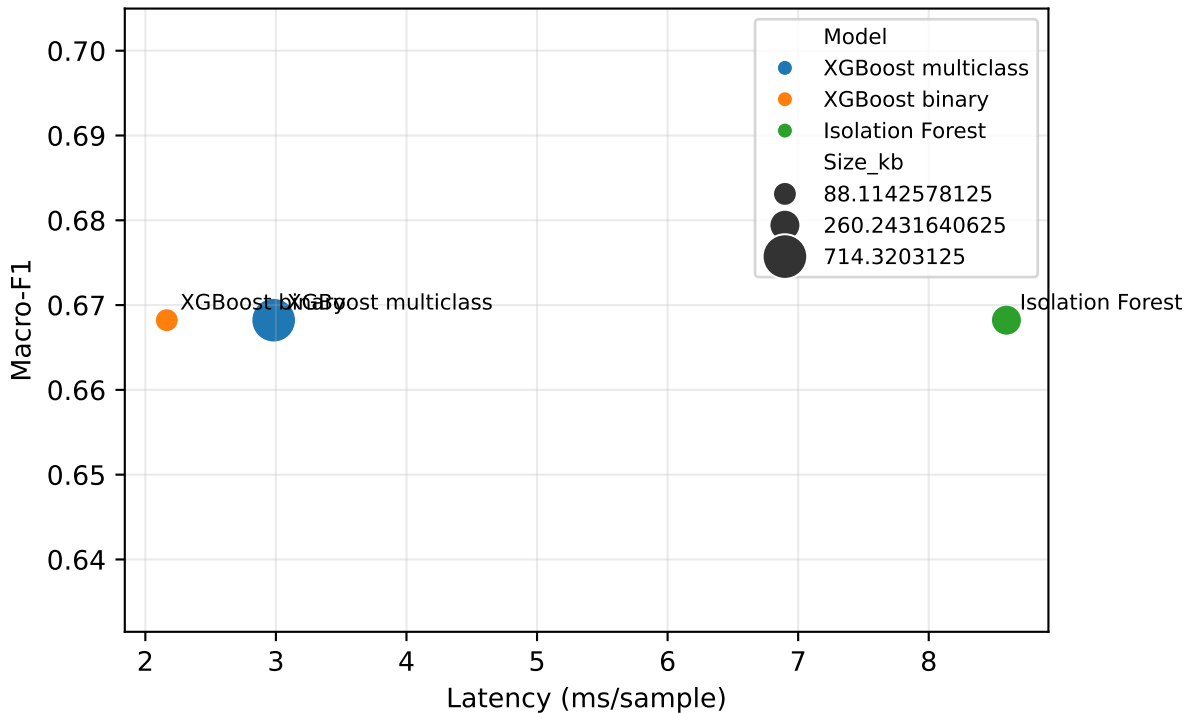
Latency vs F1
