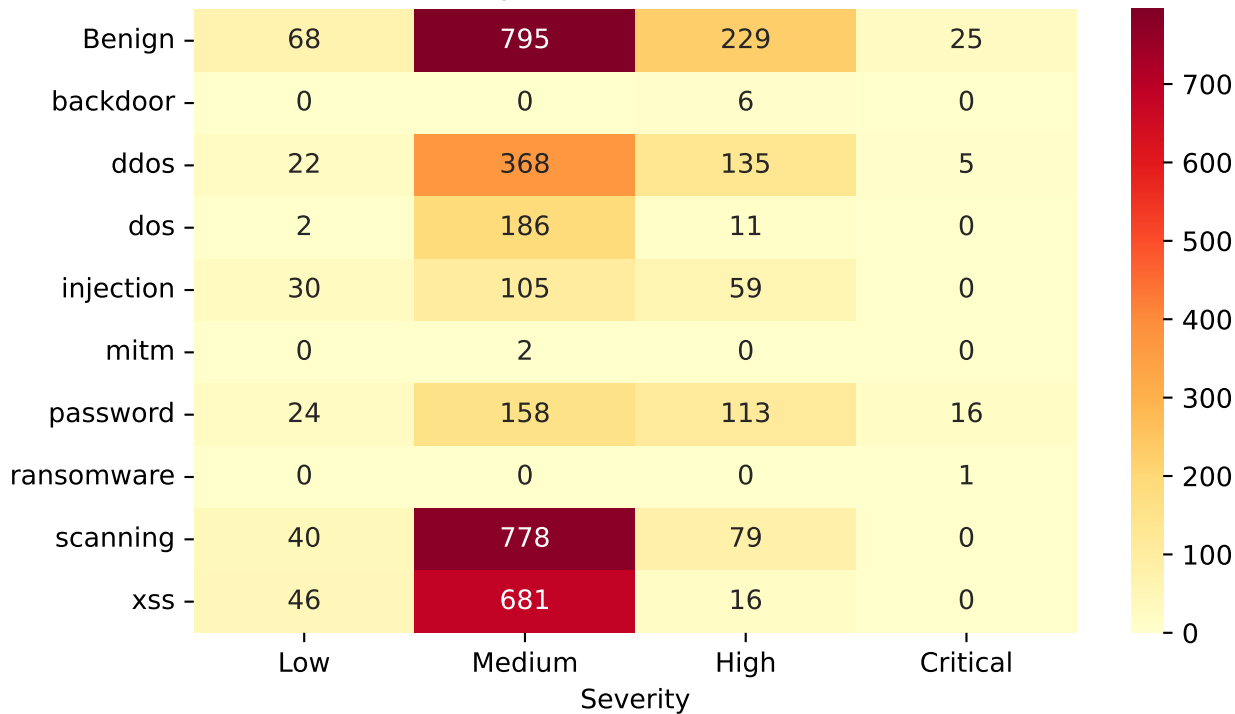
Severity vs Actual Attack Label
