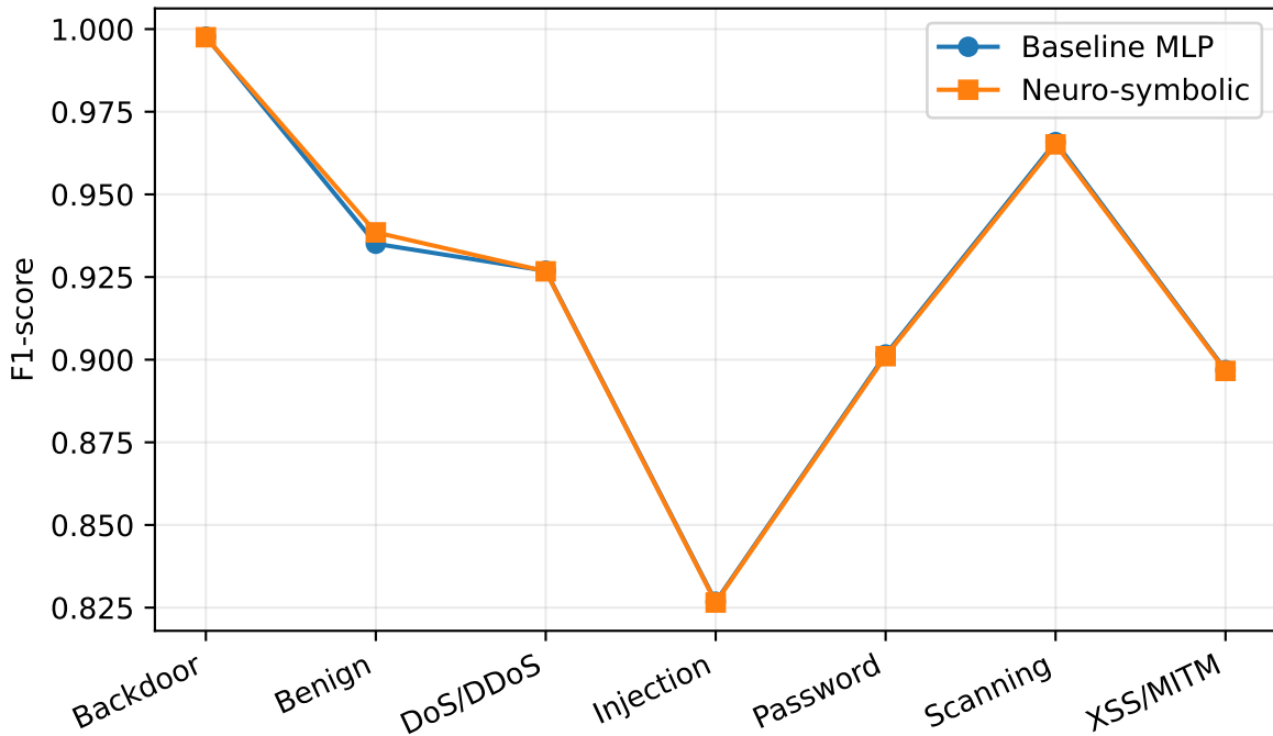
Per-Class F1 Comparison
