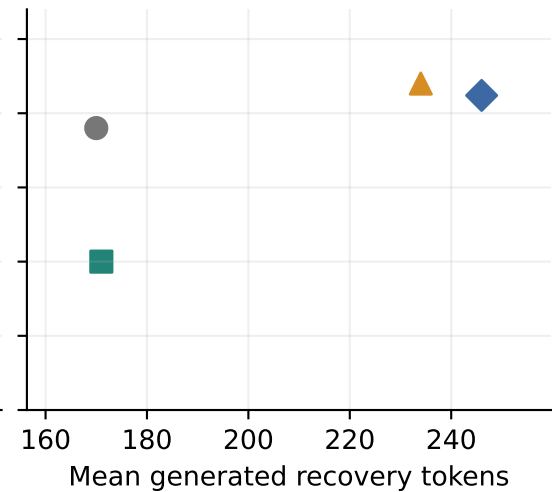
2WikiMHQA
