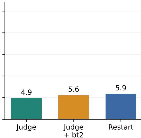
MuSiQue
