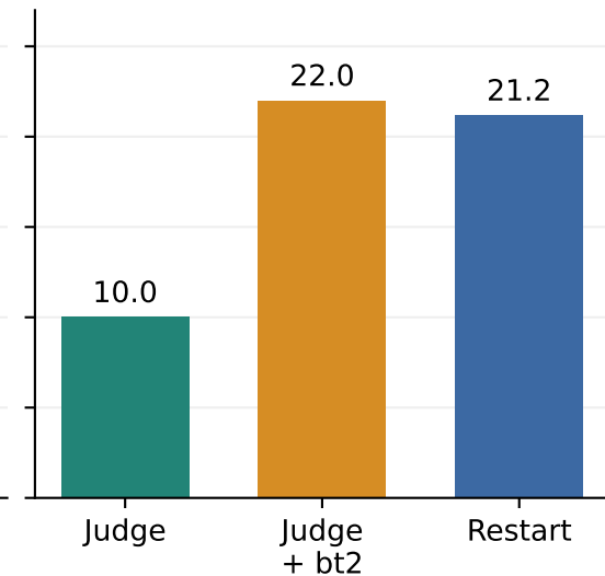
2WikiMHQA
