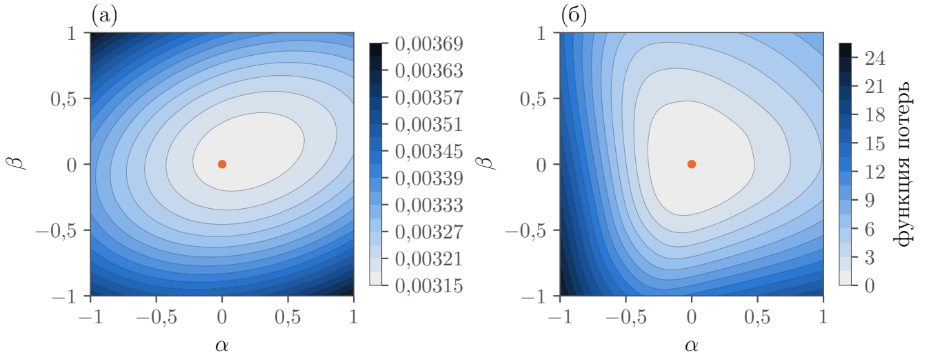
Рисунок 3.7 — Двумерные сечения функции потерь при k = 1000 на квадрате \alpha, \beta \in [-1, 1] . (а) случайные ортогональные направления, (б) два ведущих собственных вектора матрицы Гессе. Шкалы цвета различны
