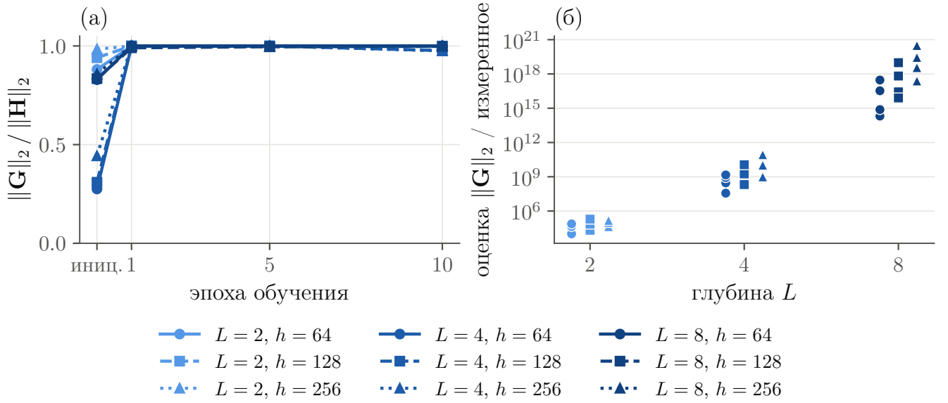
Рисунок 2.2 — Результаты для MLP: (а) отношение \|G\|_2 / \|H\|_2 в контрольных точках обучения; (б) отношение верхней оценки \|G\|_2 к измеренному значению в зависимости от глубины сети (все контрольные точки обучения)
