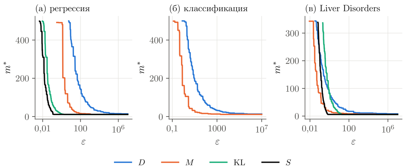
Рисунок 5.8 — Зависимость достаточного размера выборки согласно введенным критериям от гиперпараметра \varepsilon . Рассматриваются три задачи: синтетическая регрессия и классификация, а также регрессия на наборе данных Liver Disorders. Чем больше значение гиперпараметра \varepsilon , тем меньше требуется обучающих объектов
