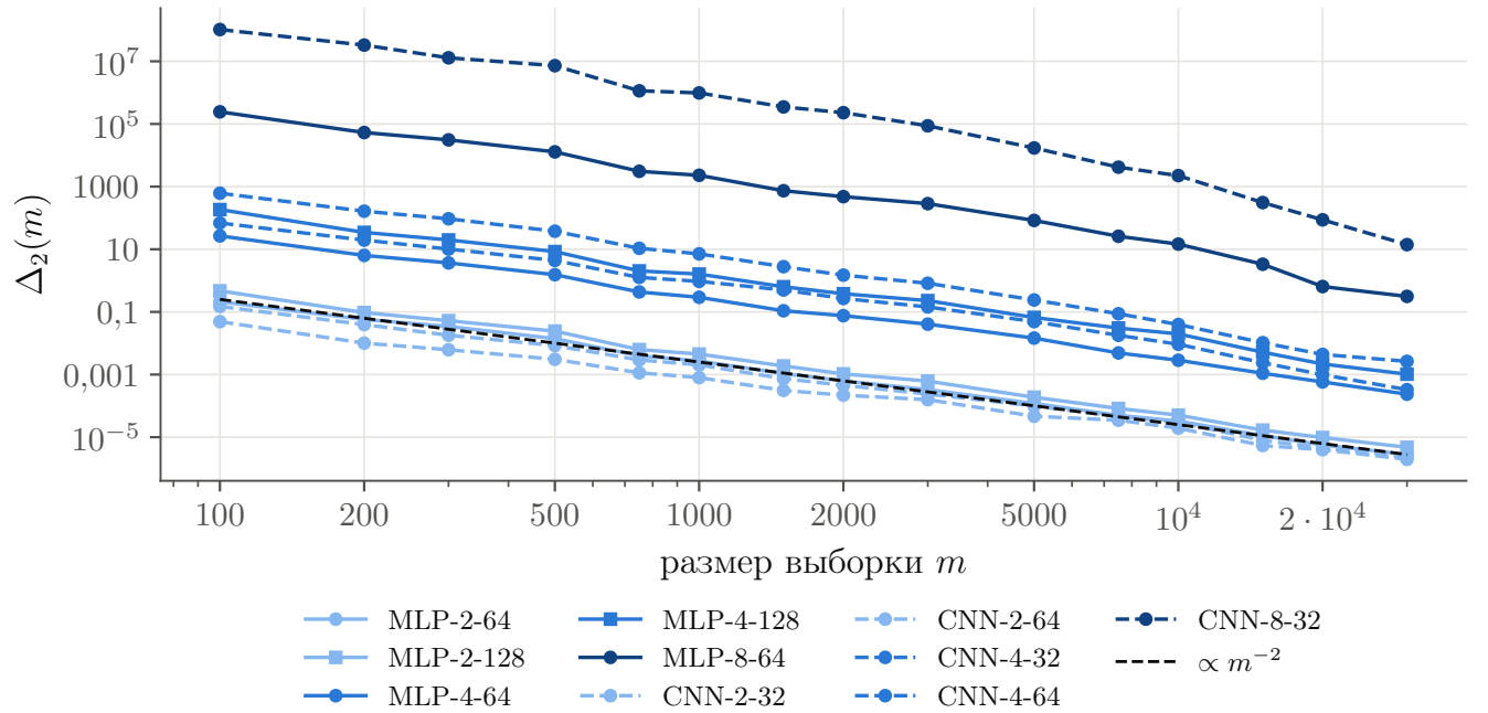
Рисунок 4.3 — Сходимость критерия \Delta_2(m) для различных архитектур. Штриховая линия имеет наклон -2 и проходит через одну точку; это порядок из тождества усреднения, а не подобранный показатель
