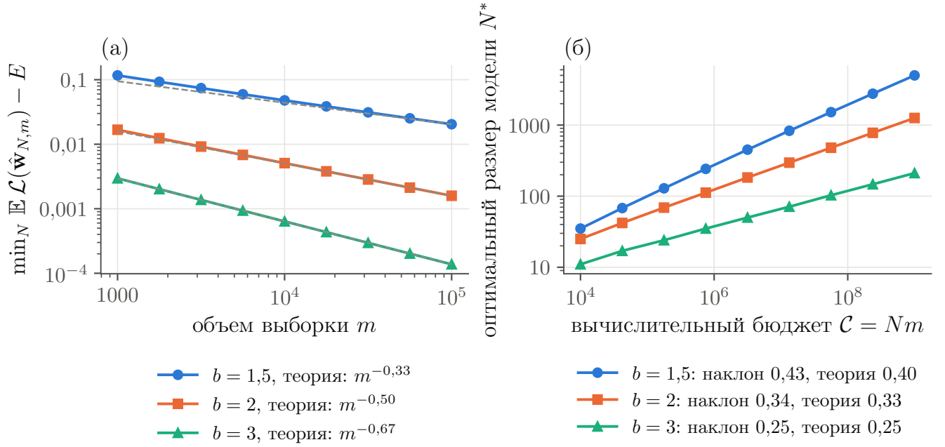
Рисунок 4.2 — Показатели закона масштабирования в модели с неполным набором признаков ( D = 10^6 , \lambda_j = j^{-1.5} ): (а) риск при оптимальном размере модели в зависимости от объема данных для трех значений b , штриховые линии — теоретический наклон -(b-1)/b ; (б) вычислительно-оптимальный размер модели в зависимости от бюджета C = Nm и его наклон в сравнении с теоретическим значением 1/(b+1)
