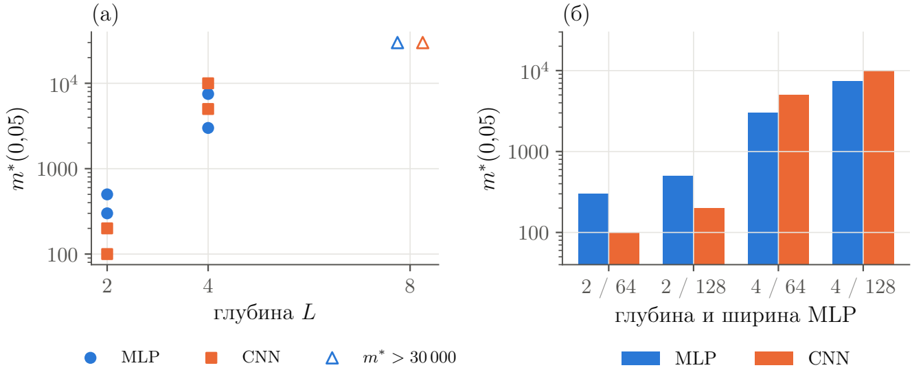
Рисунок 4.4 — Влияние глубины на достаточный размер выборки при \varepsilon = 0,05 . Слева: m^* для MLP и CNN; пустой треугольник — порог не достигнут до 30 000. Справа: пары одной глубины, подпись — глубина и ширина MLP
