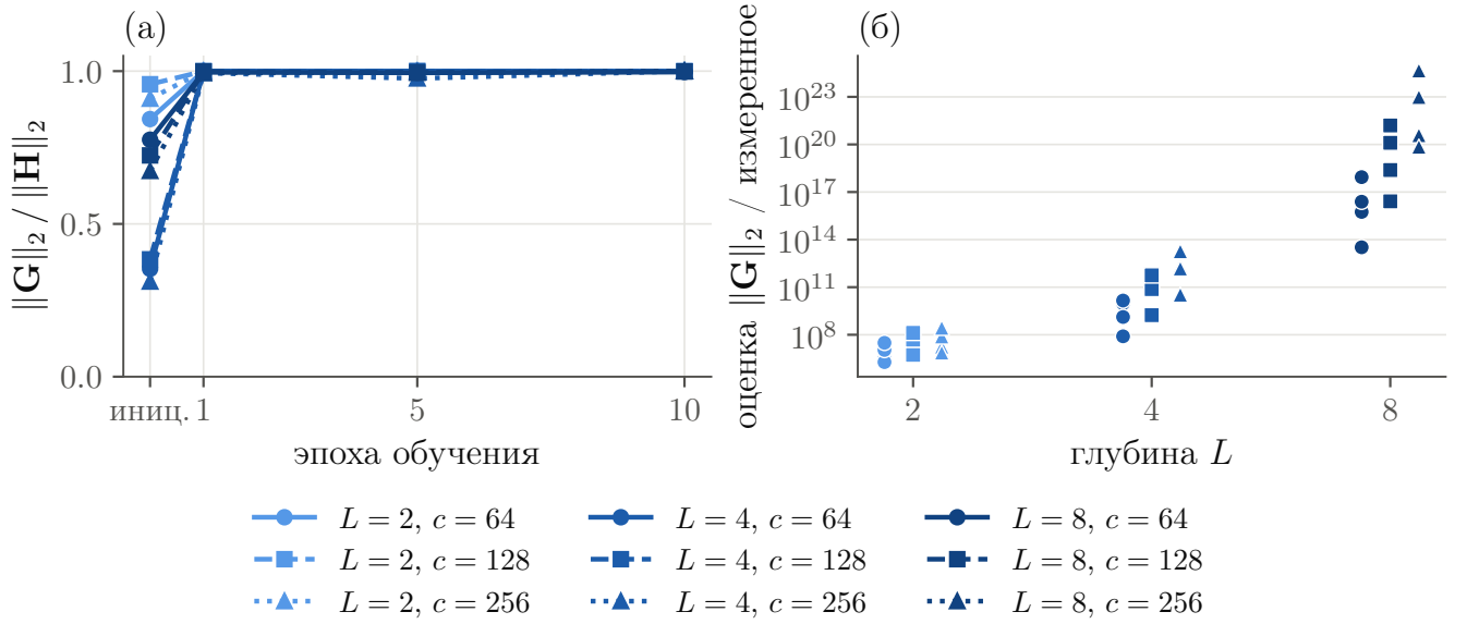
Рисунок 2.3 — Результаты для CNN: (а) отношение \|G\|_2 / \|H\|_2 в контрольных точках обучения (значения ограничены отрезком [0, 1] ); (б) отношение верхней оценки \|G\|_2 к измеренному значению в зависимости от глубины сети
