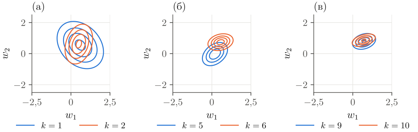
Рисунок 5.4 — Изменение апостериорных распределений параметров на схожих подвыборках по мере увеличения их размера. Двумерный случай, где на графиках изображены линии уровня
