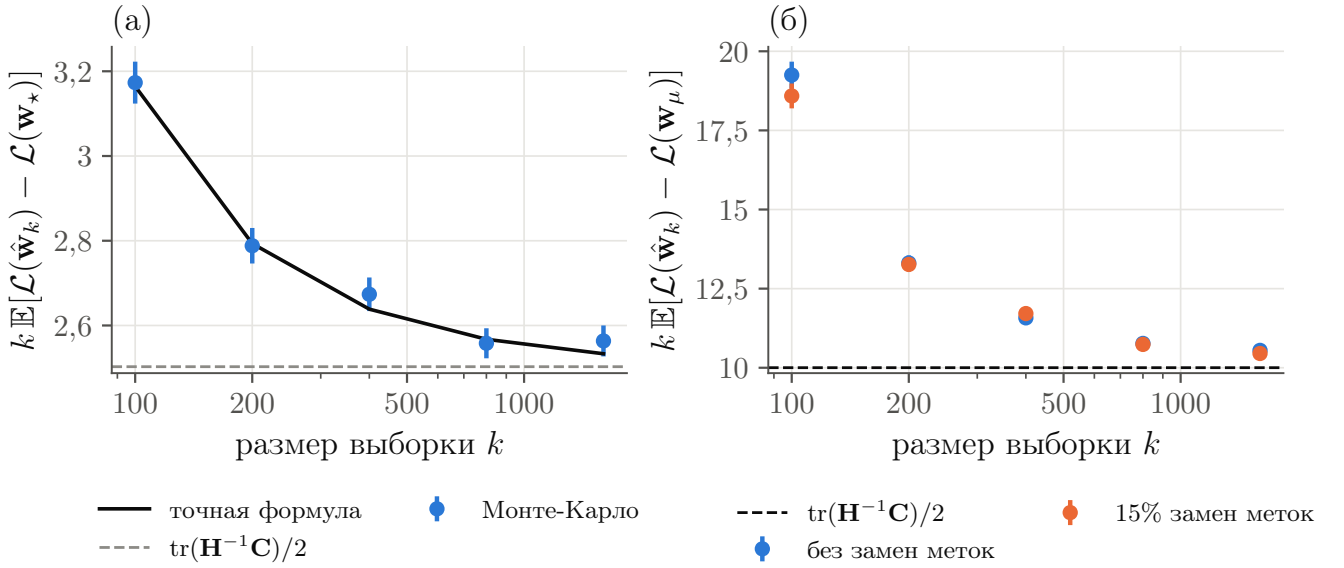
Рисунок 4.6 — Локальный режим, n = 20 , 2 000 повторений, отрезки — две стандартные ошибки. (а) Линейная регрессия: точки — Монте-Карло, сплошная линия — точная формула, штриховая — \text{tr}(\mathbf{H}^{-1}\mathbf{C})/2 . (б) Логистическая регрессия с верными метками и с заменой 15% меток; штриховая линия — та же константа по популяционному спектру
