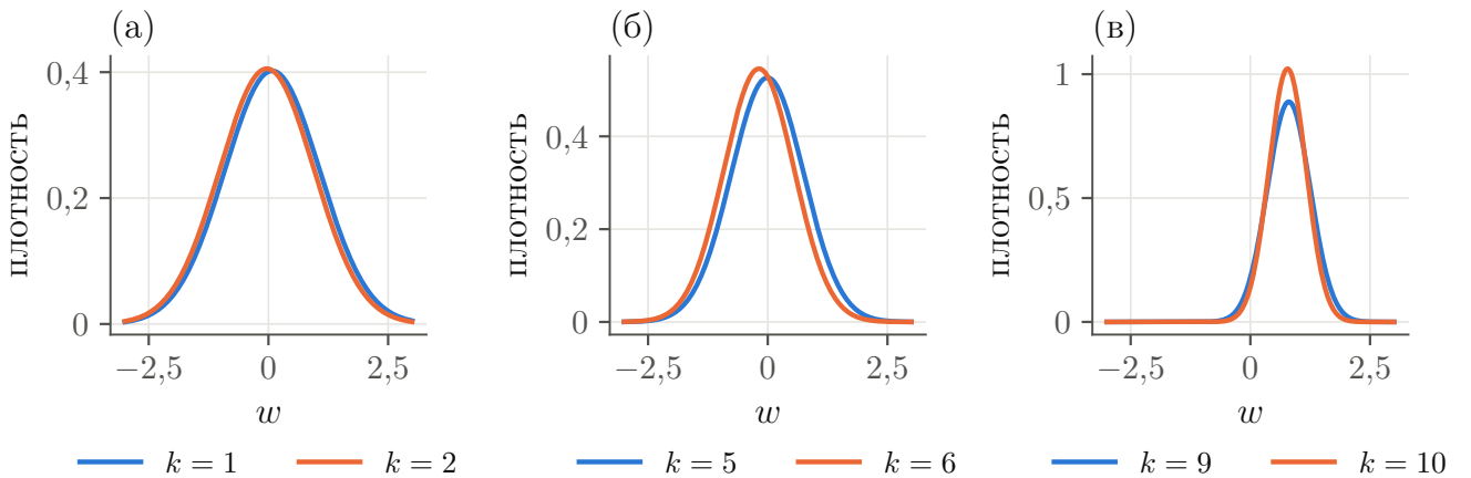
Рисунок 5.3 — Изменение апостериорных распределений параметров на схожих подвыборках по мере увеличения их размера. Одномерный случай, где на графиках изображены плотности распределений
