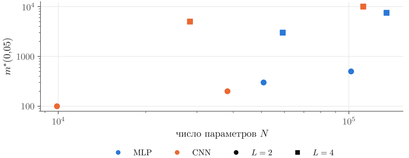
Рисунок 4.5 — Достаточный размер выборки m^*(\varepsilon) в зависимости от числа параметров для MLP и CNN
