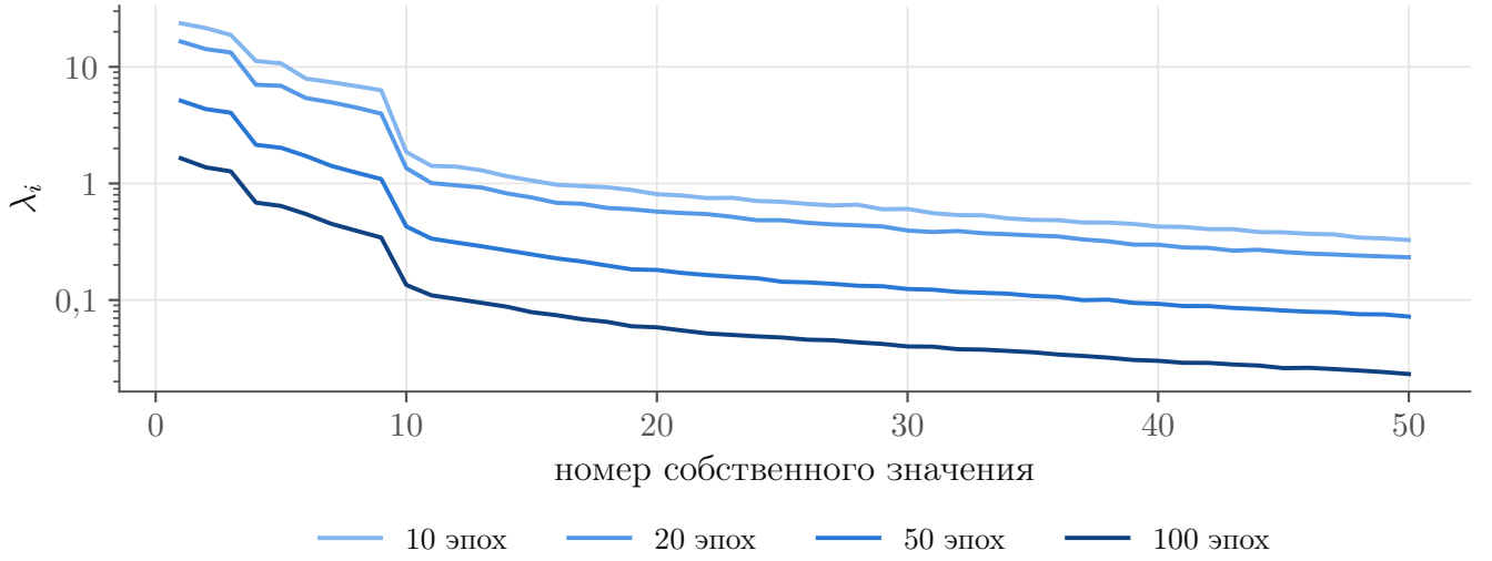
Рисунок 3.6 — Ведущие собственные значения матрицы Гессе на разных эпохах обучения. После первых номеров убывание становится более пологим, масштаб спектра падает с числом эпох
