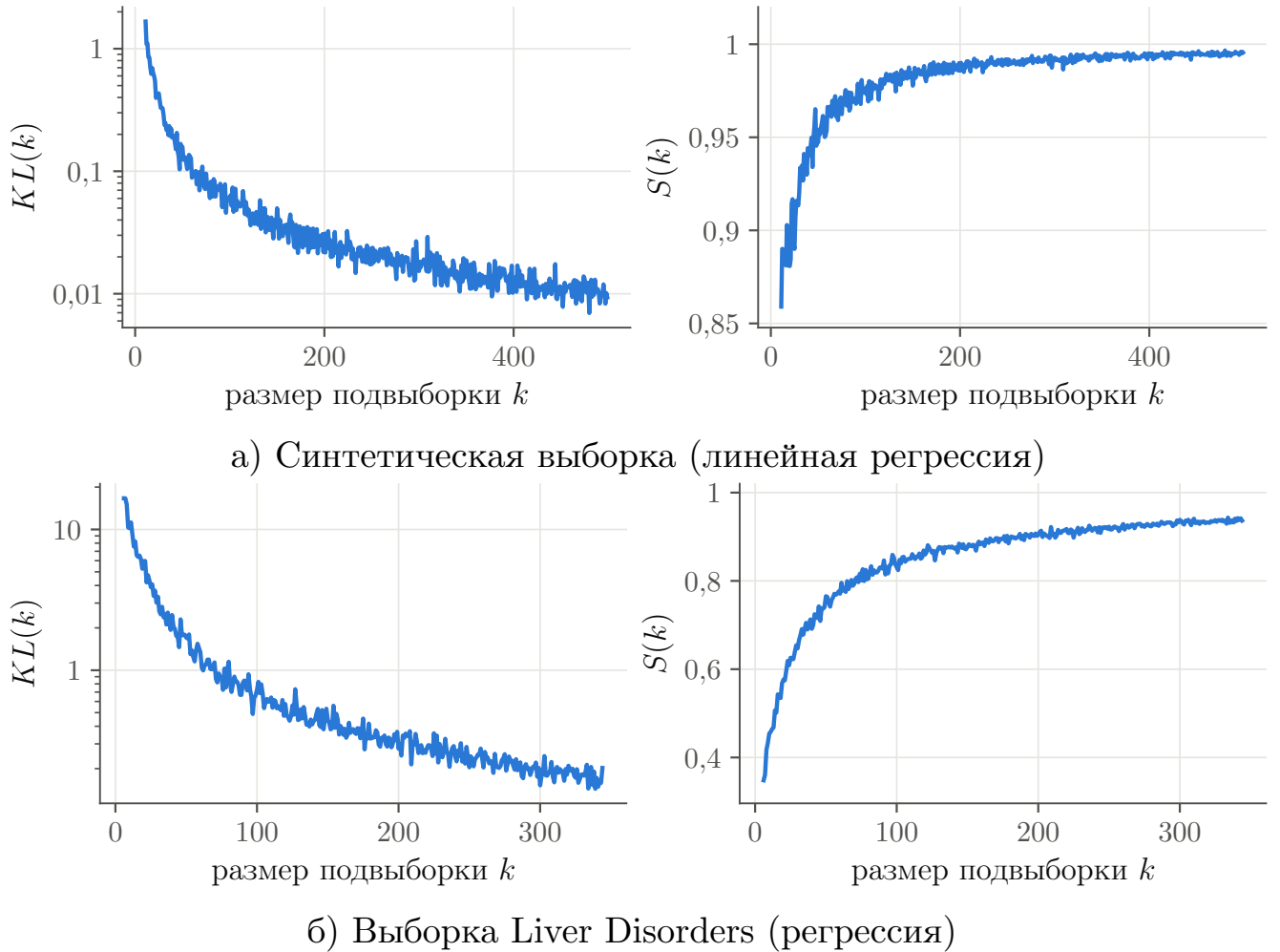
Рисунок 5.7 — Сходимость функций KL(k) и S(k) в различных задачах и на различных выборках. Оба критерия стремятся к предельным значениям при увеличении размера выборки
