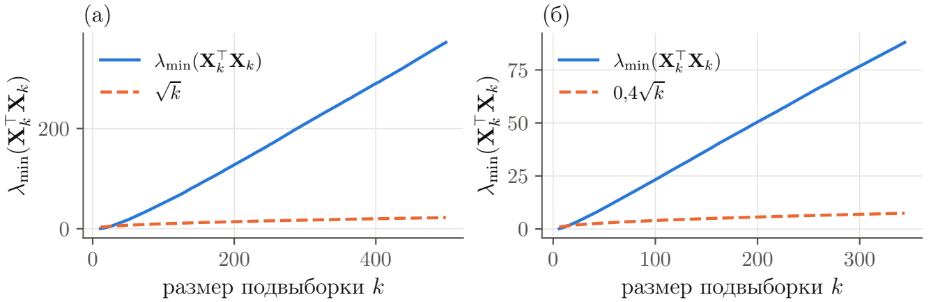
Рисунок 5.6 — Изменение минимального собственного значения матрицы \mathbf{X}_k^T \mathbf{X}_k при увеличении размера выборки в задачах синтетической линейной регрессии и регрессии на наборе данных Liver Disorders
