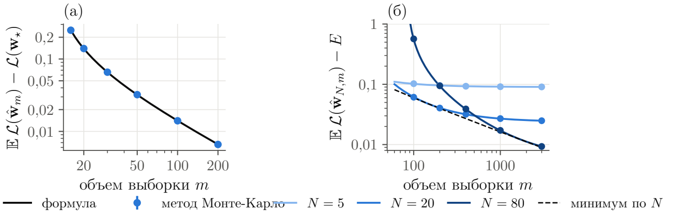
Рисунок 4.1 — Точно решаемые модели: (а) средний избыточный риск метода наименьших квадратов при n = 10 и формула (4.13); (б) средний риск модели с N признаками при \lambda_j = j^{-1,5} , e_j = j^{-2} , \sigma = 0,5 и формула (4.17); штриховая линия — минимум по N . Точки — метод Монте-Карло, отрезки — две стандартные ошибки
