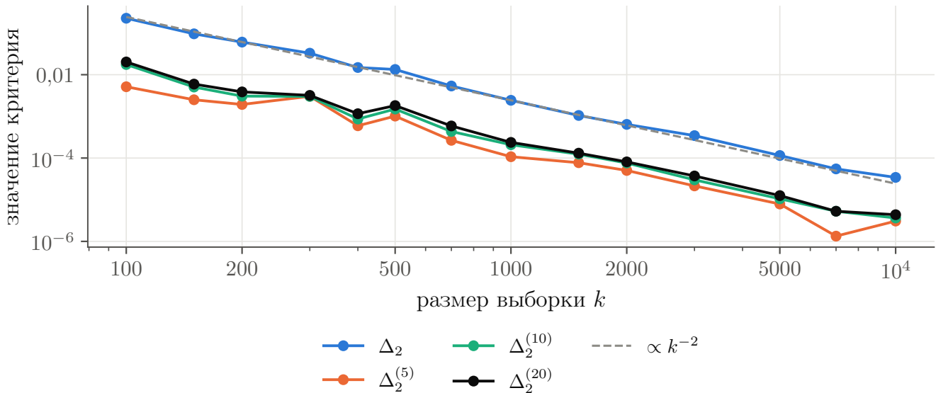
Рисунок 3.5 — Среднеквадратичный критерий \Delta_2(k) и его сужения на D = 5, 10, 20 ведущих собственных направлений. Штриховая линия — пропорциональность k^{-2}
