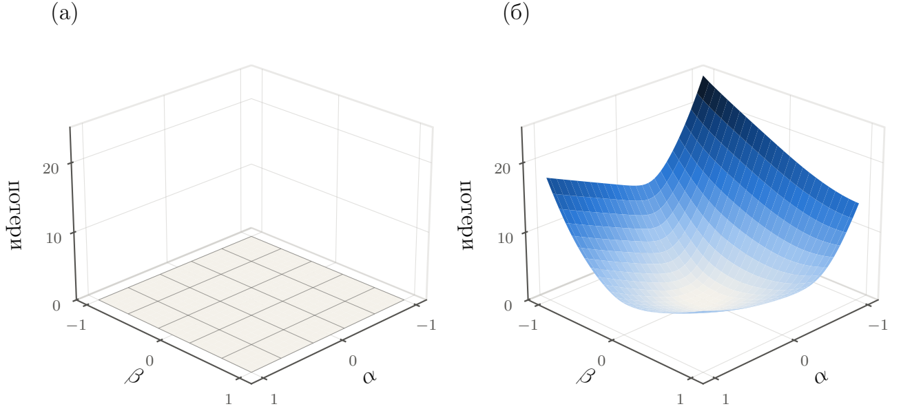
Рисунок 3.8 — Те же сечения и тот же квадрат. Вертикальная ось общая: панель (а) остается плоскостью, панель (б) поднимается вдоль ведущих собственных направлений
