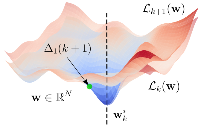
Рисунок 3.2 — Иллюстрация абсолютного однотоочечного критерия сходимости \Delta_1(k)
