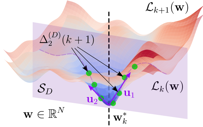
Рисунок 3.4 — Иллюстрация среднеквадратичного критерия сходимости в подпространстве наибольшей кривизны \Delta_2^{(D)}(k)
