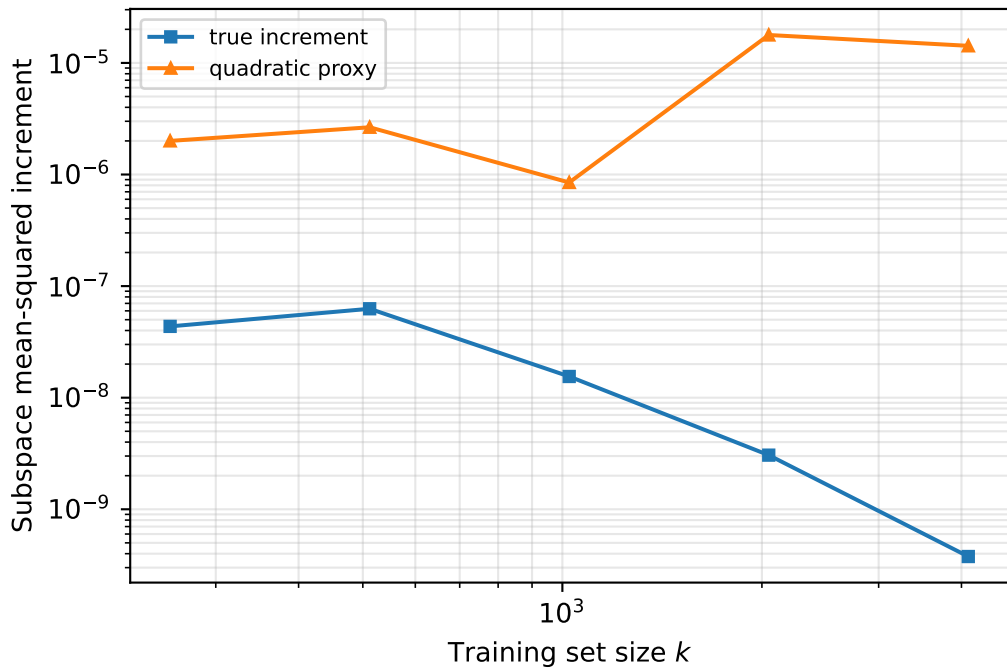
wikitext2 medium
