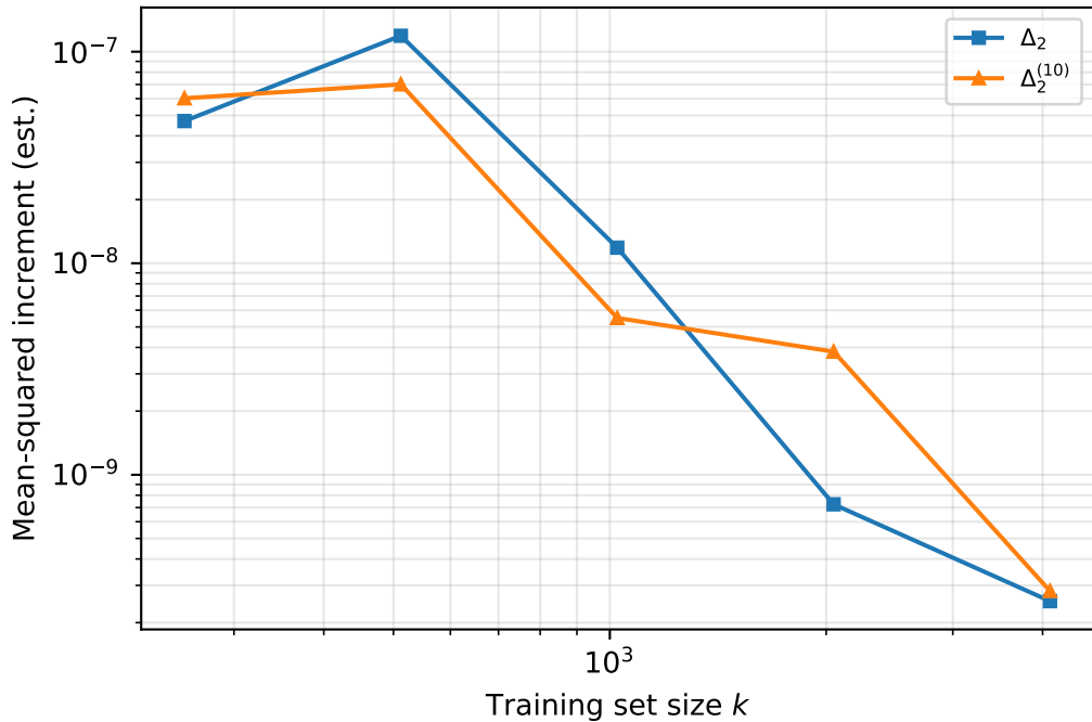
wikitext2 medium (D=10)
