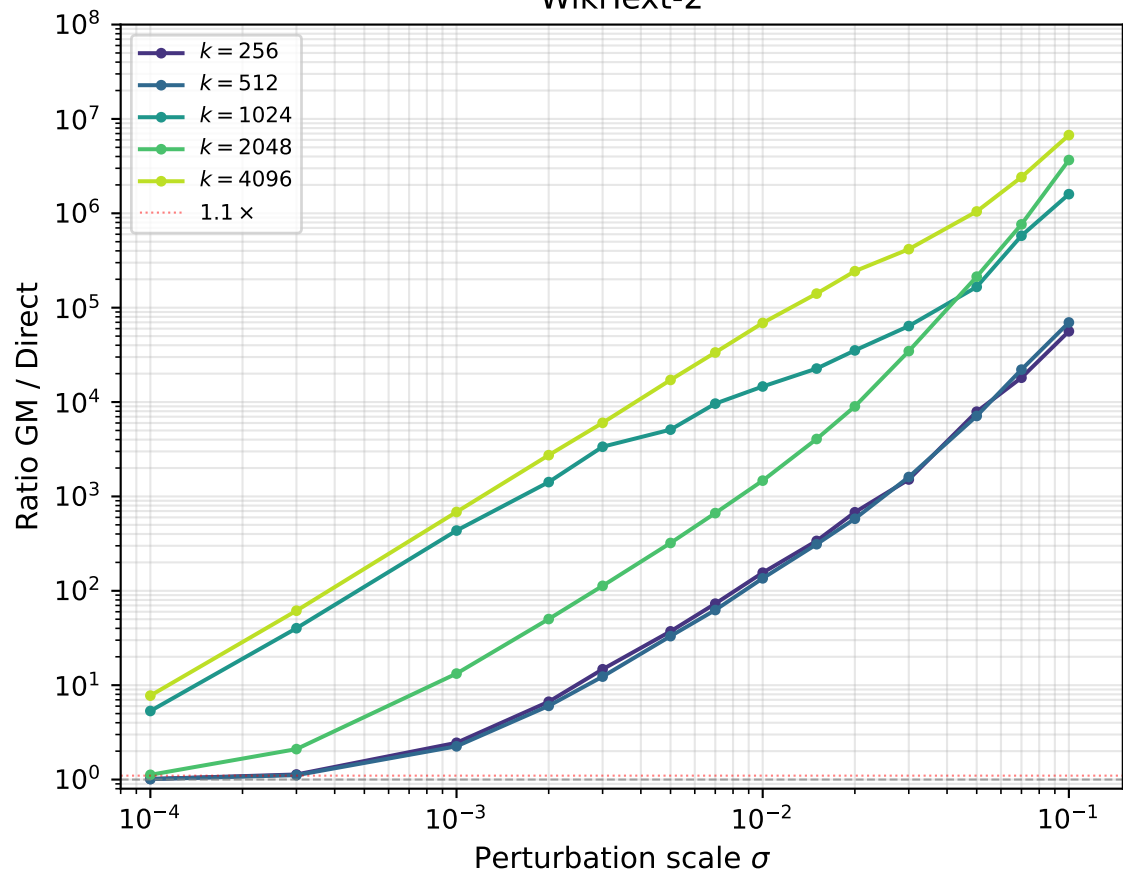
WikiText-2
