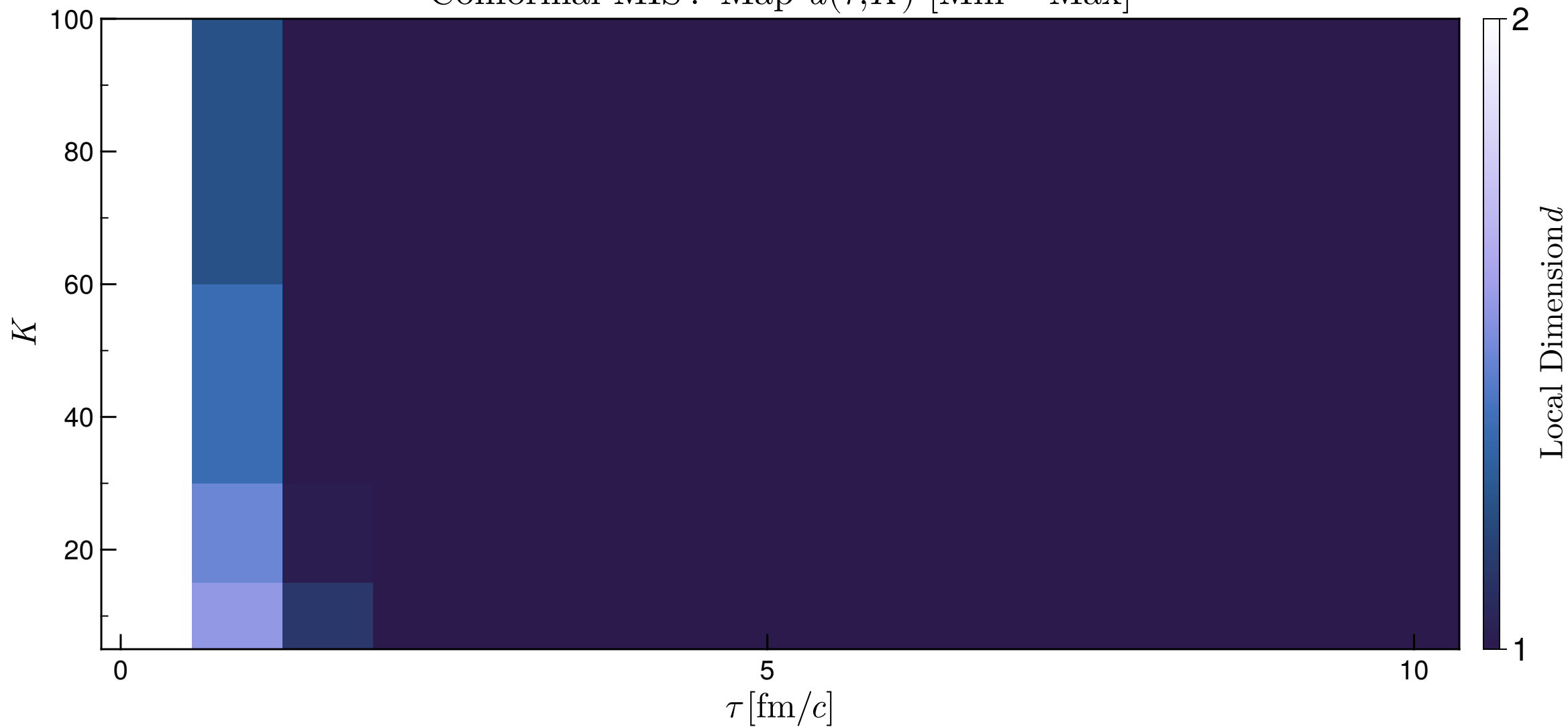
Conformal MIS : Map d(\tau, K) [Min – Max]
