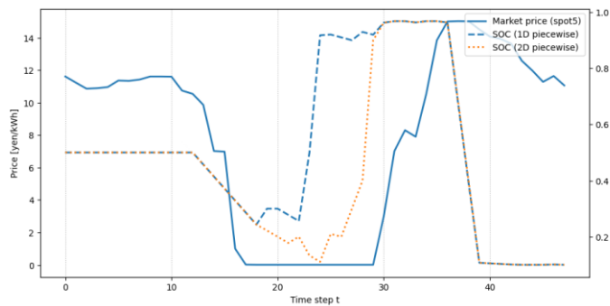
図 7 5 月における 1 次元、2 次元のピースワイズ劣化を考慮した SOC と市場価格
