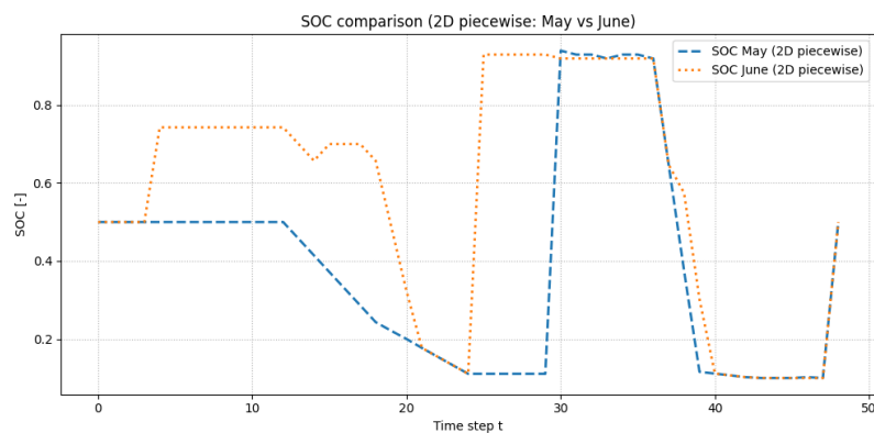
図 4 5月と6月のSOC推移
