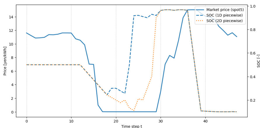
図 7 5 月における一次元，二次元のピースワイズ劣化を考慮した SOC と市場価格
