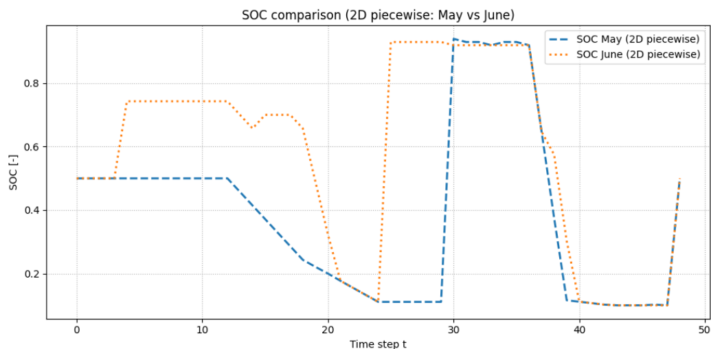
図 4 5月と6月の SOC 推移
