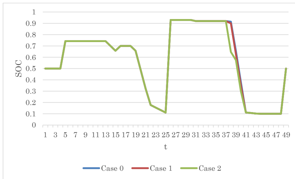
図 8 6月における SOC 偏移
