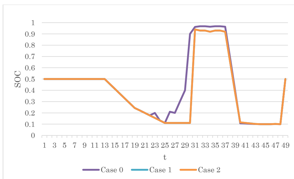
図 5 5 月における SOC 偏移
