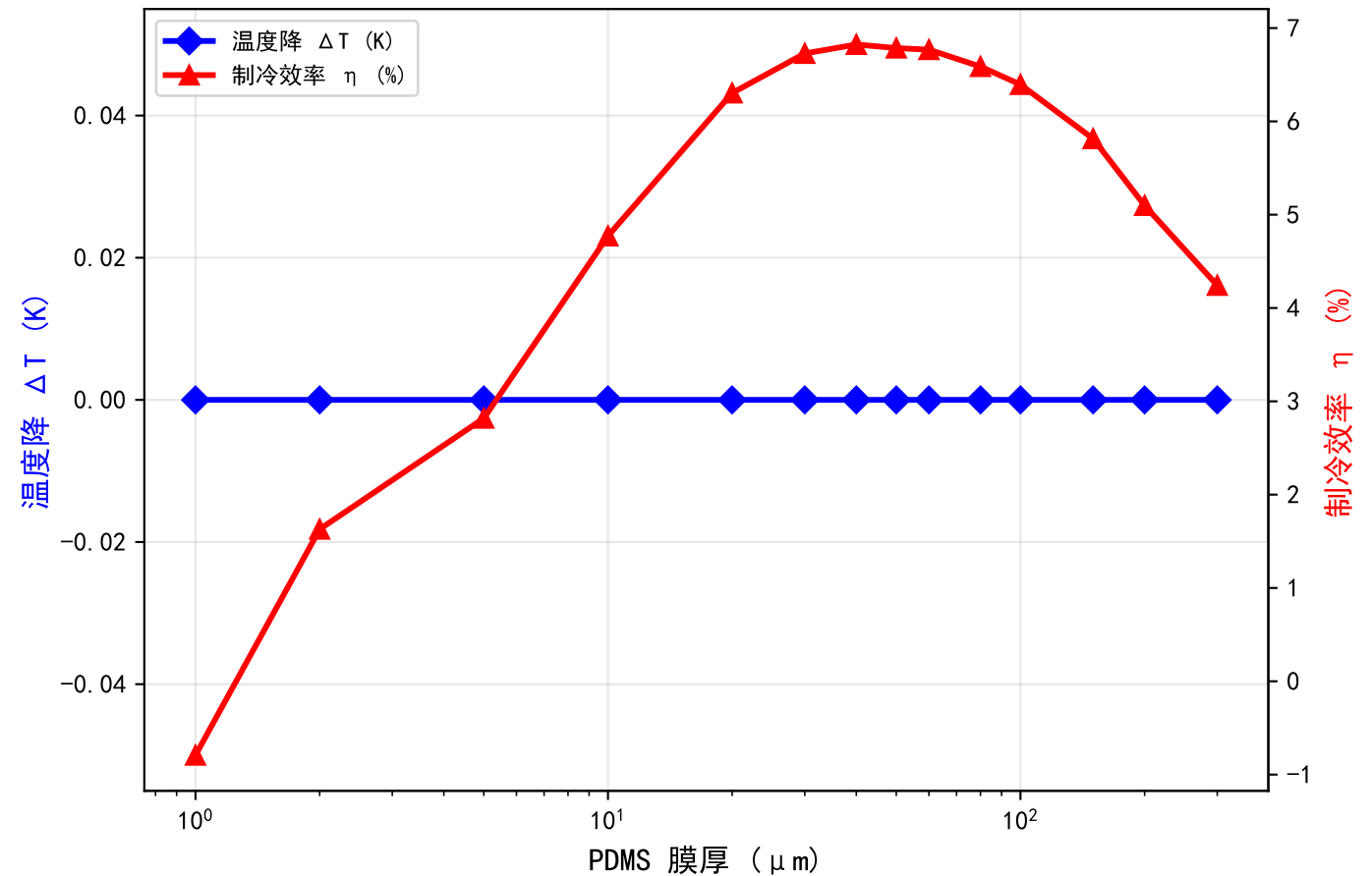
稳态温度降与制冷效率
