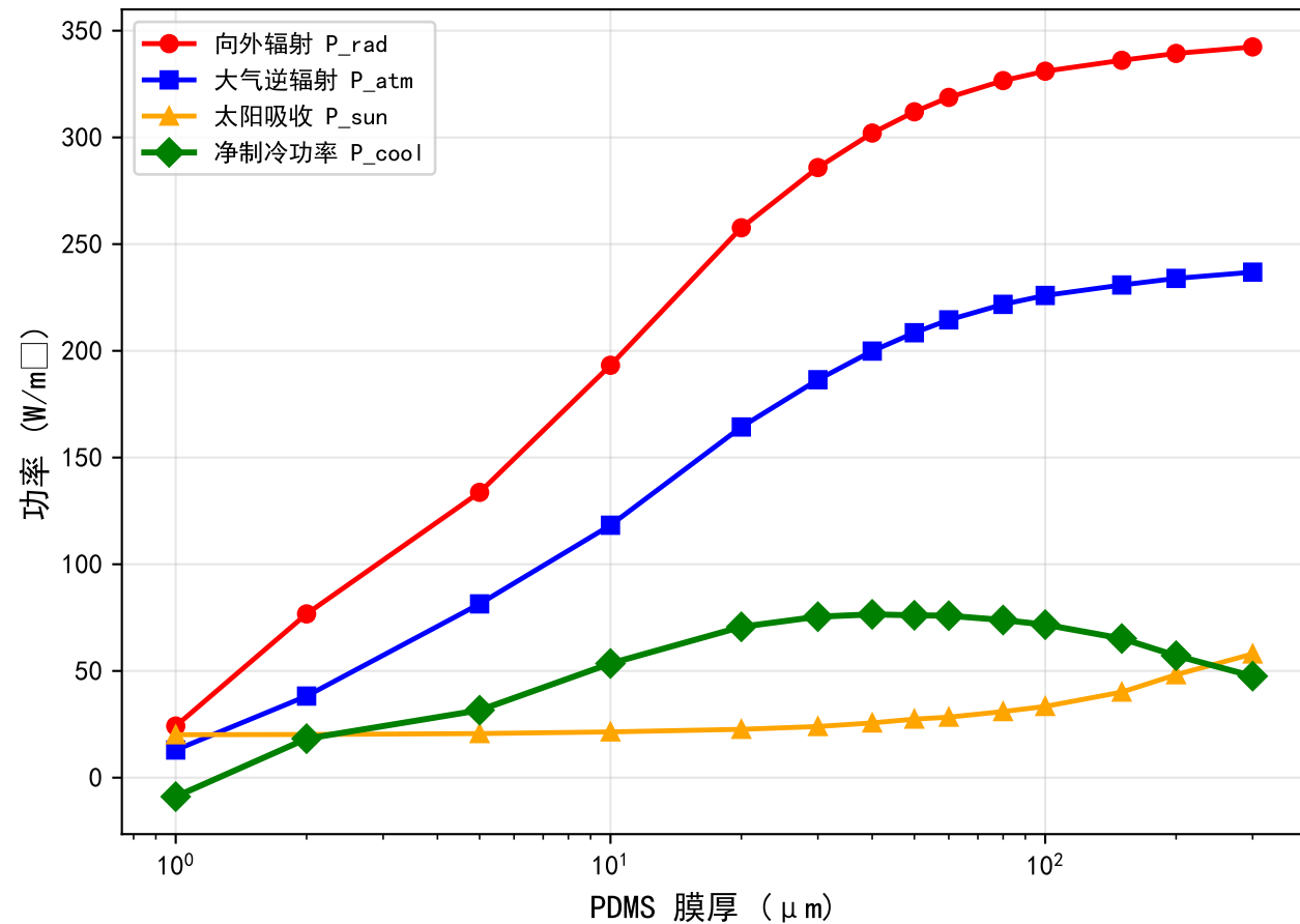
辐射制冷各分量随膜厚变化
