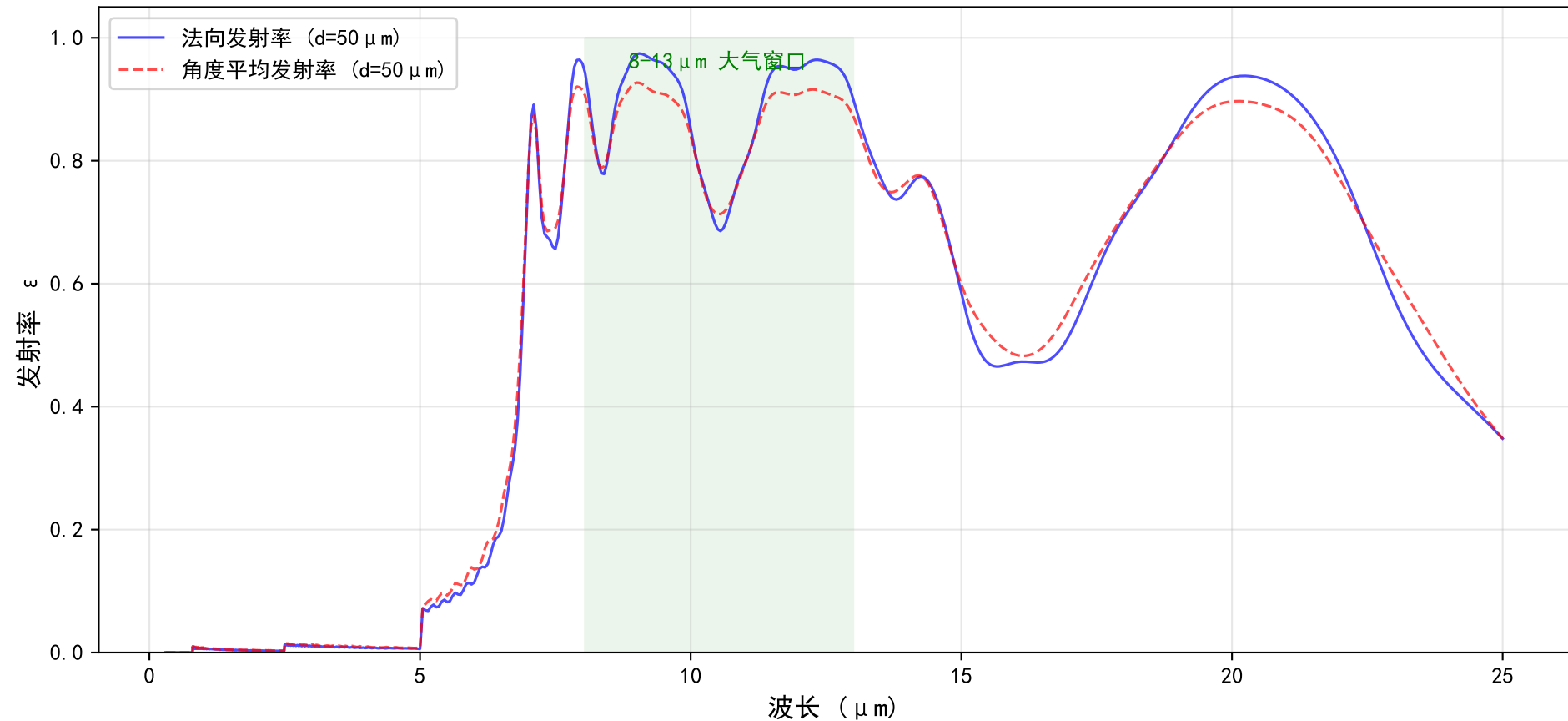
法向发射率与角度平均发射率对比
