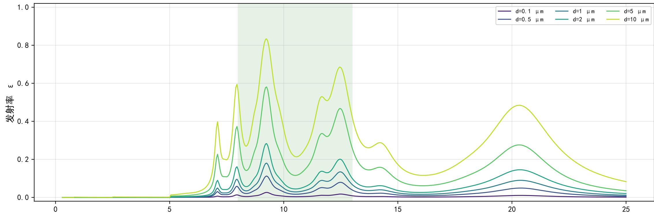
不同厚度 PDMS 薄膜的光谱发射率 \varepsilon(\lambda) — 法向入射
