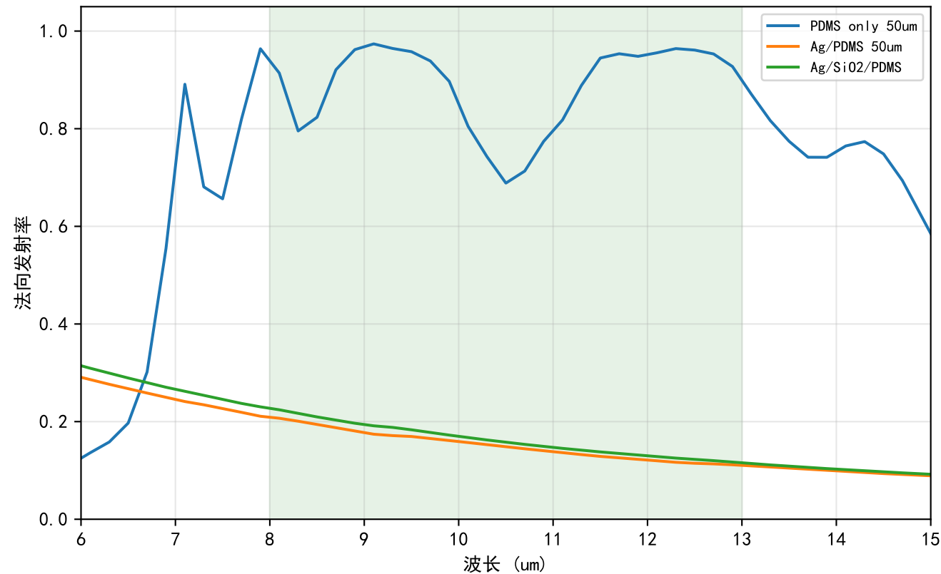
8-13um IR发射率光谱
