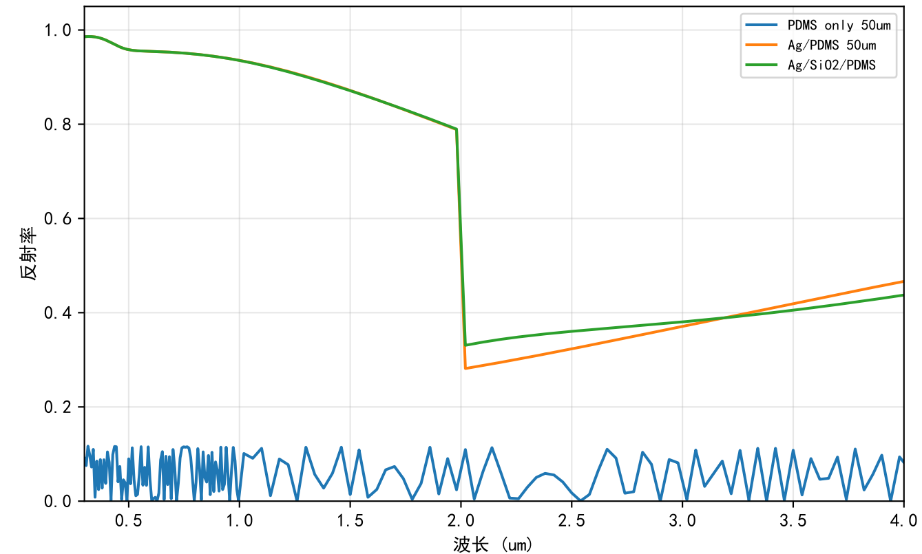
太阳波段反射率
