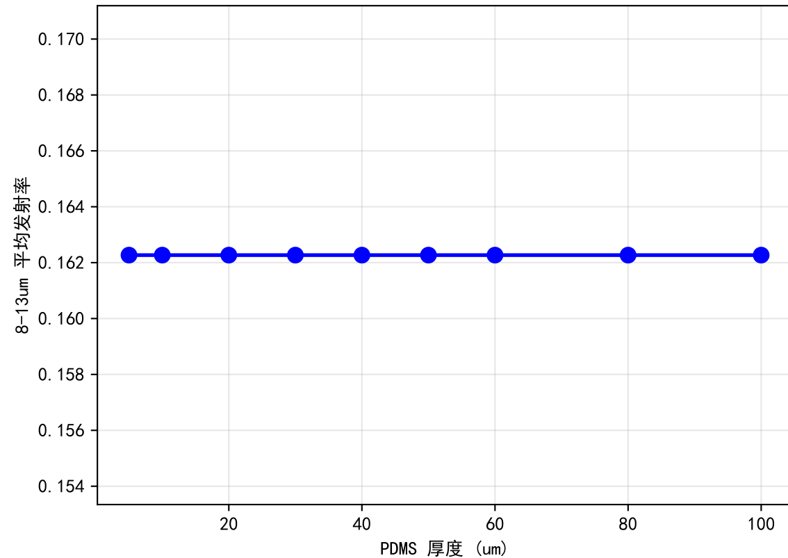
PDMS厚度对IR发射率的影响
