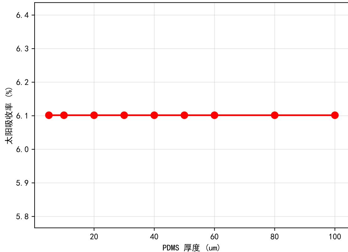
PDMS厚度对太阳吸收的影响
