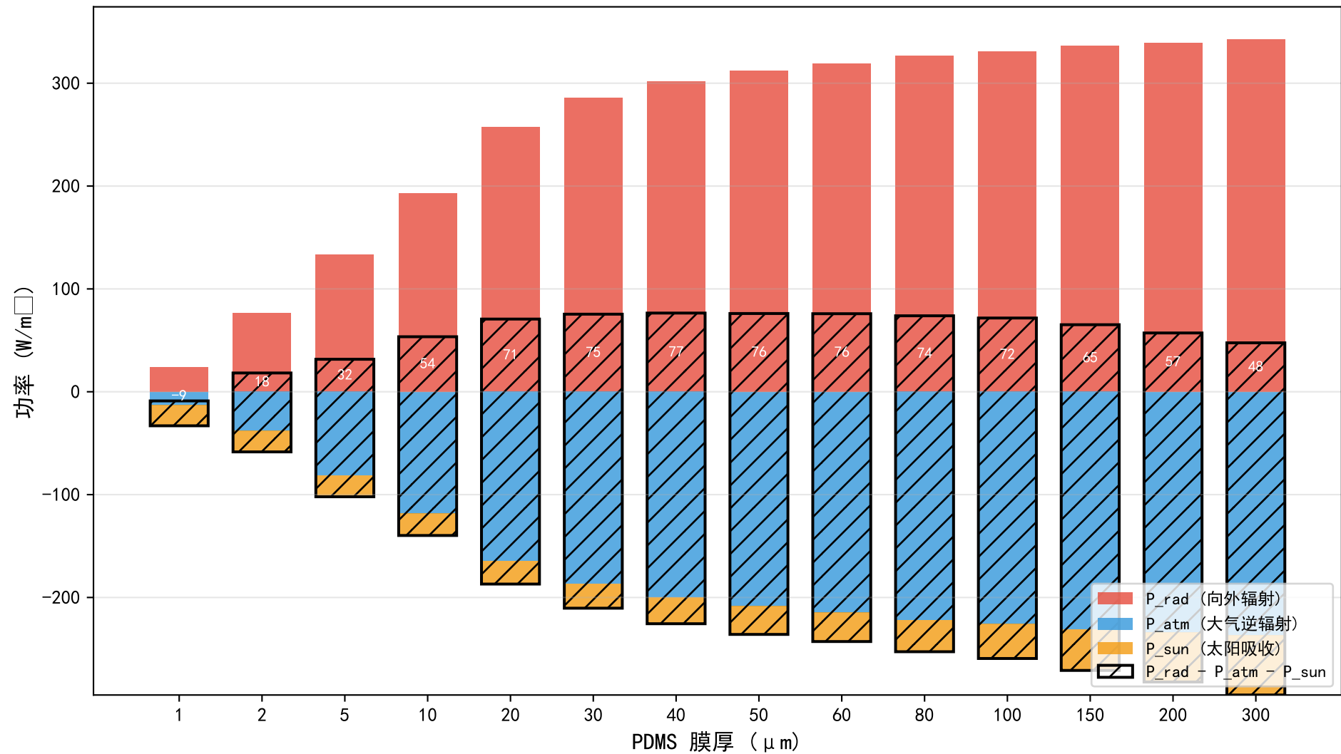
辐射制冷各分量随膜厚变化
