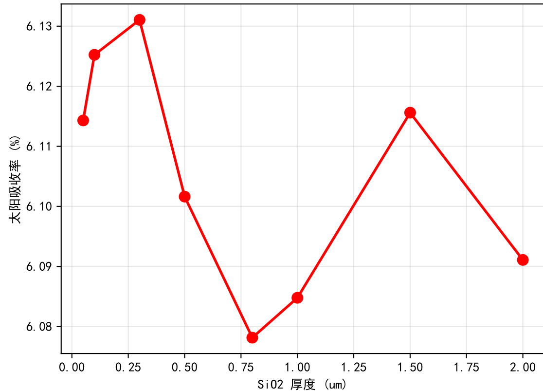
SiO 2 厚度对太阳吸收的影响
