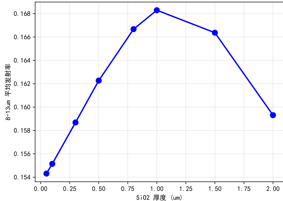
SiO 2 厚度对IR发射率的影响
