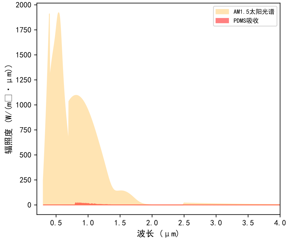
太阳光谱与PDMS太阳吸收
