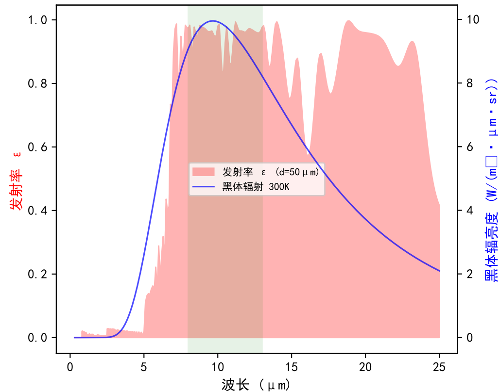
发射率与300K黑体辐射
