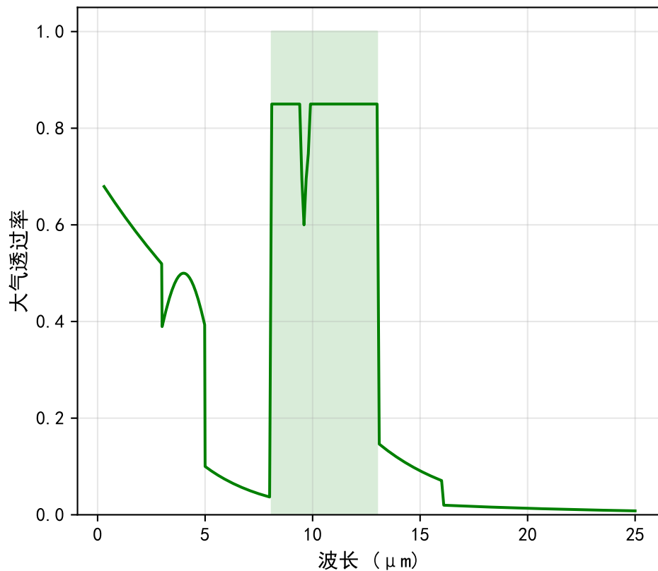
大气透过率光谱 (8-13 \mu\text{m} 窗口)
