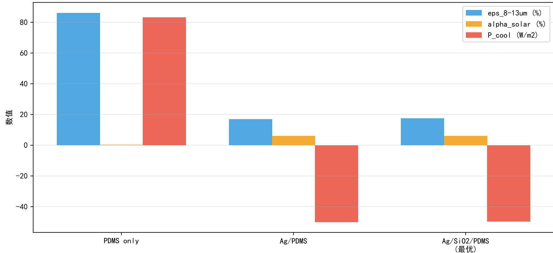
多层膜结构设计对比
