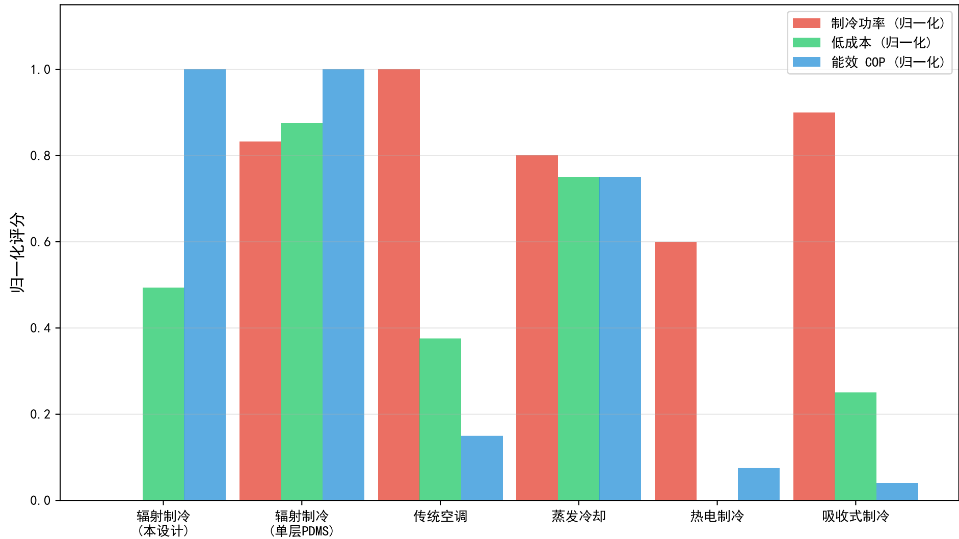
辐射制冷与其他制冷技术对比
