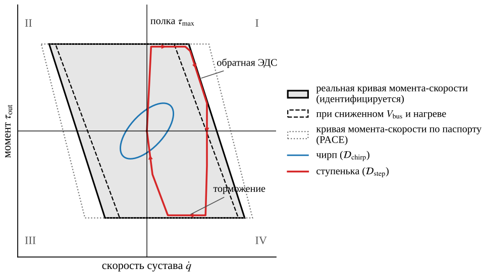
Рисунок 2.1 – Кривая момента-скорости и пример траекторий (I–IV — квадранты, величины условные)
