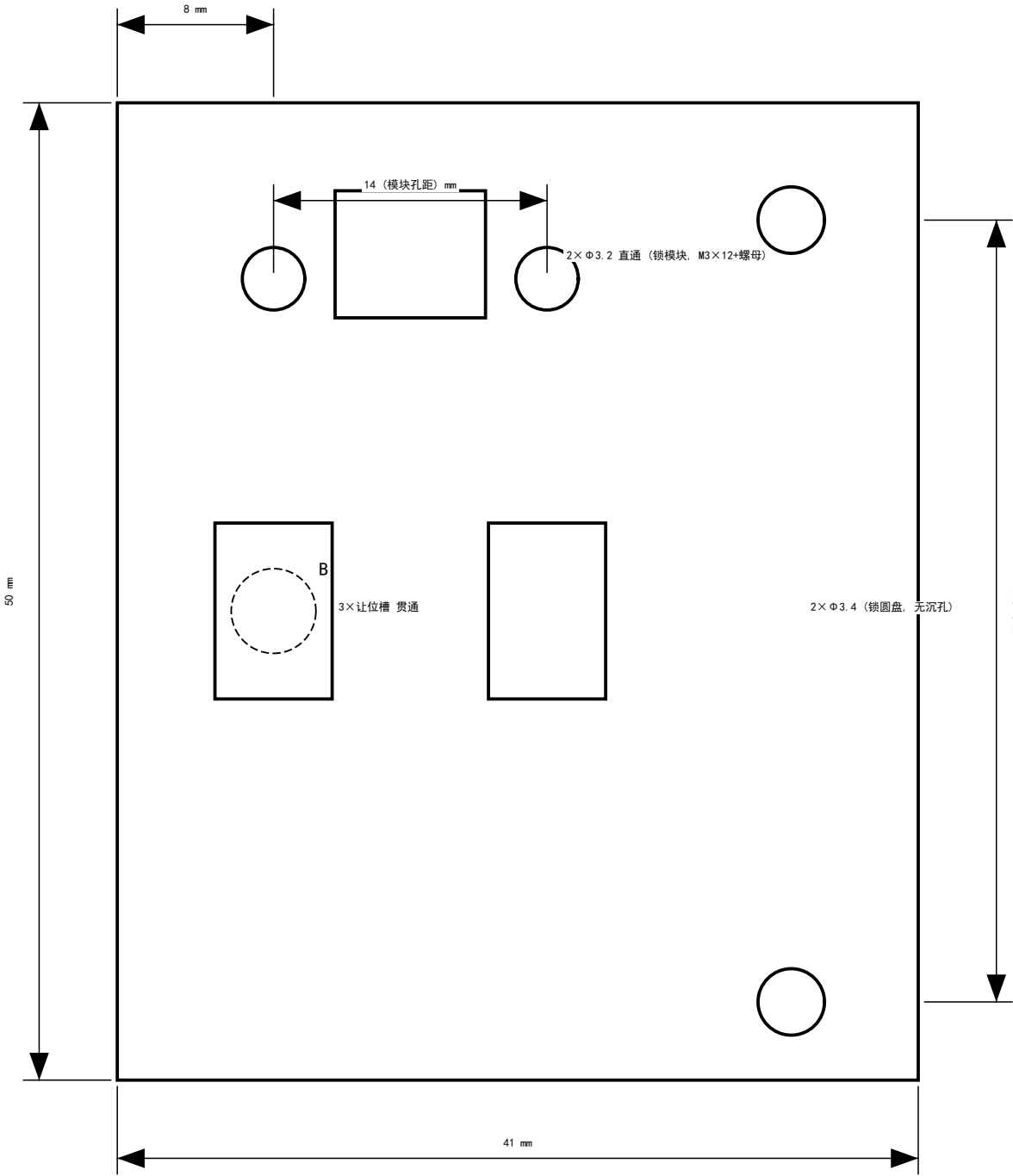
俯视 (3:1) （沿 -Z 看顶面） 尺寸单位：mm
