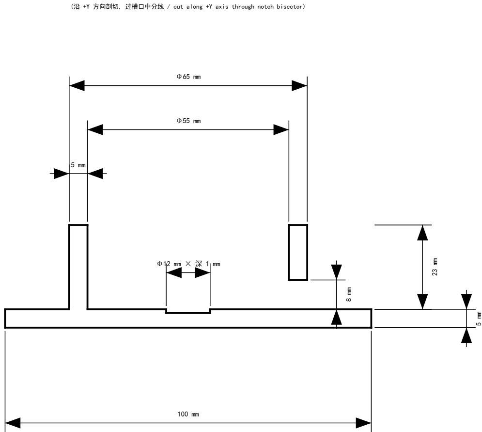
剖视图 Section A-A (1:1) 尺寸单位: mm
