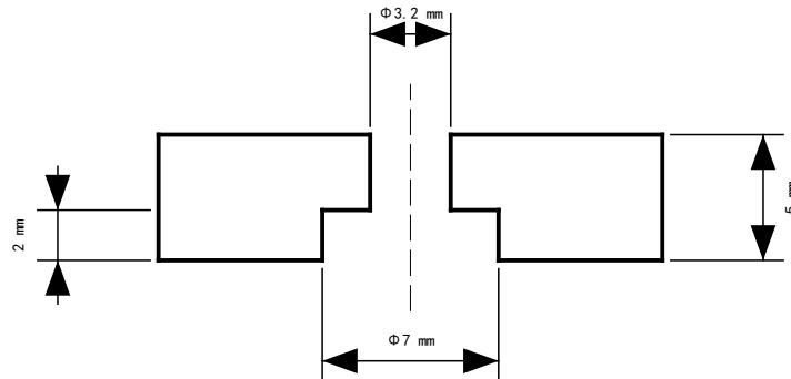
详图 B Detail B (3:1) 尺寸单位: mm
