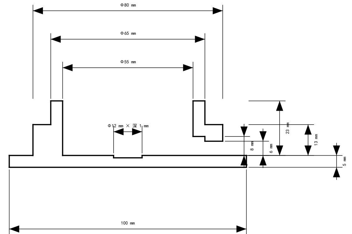
详图 B Detail B (3:1) 尺寸单位: mm
