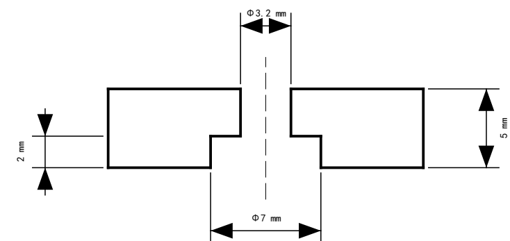
详图 B Detail B (3:1) 尺寸单位: mm
