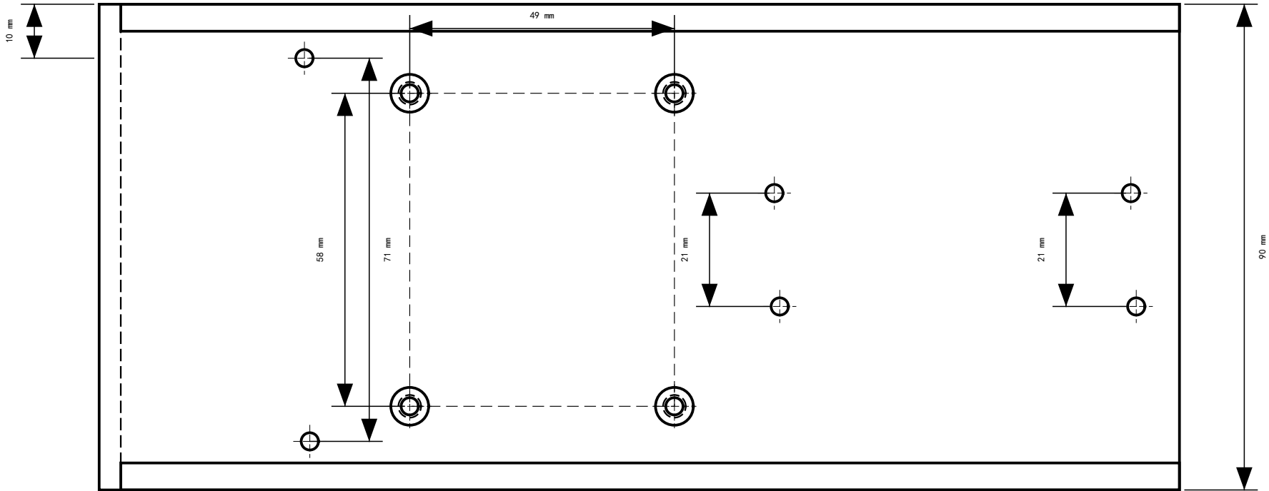
俯视图 Top View (1:1) 尺寸单位: mm (沿 -Z 看)
