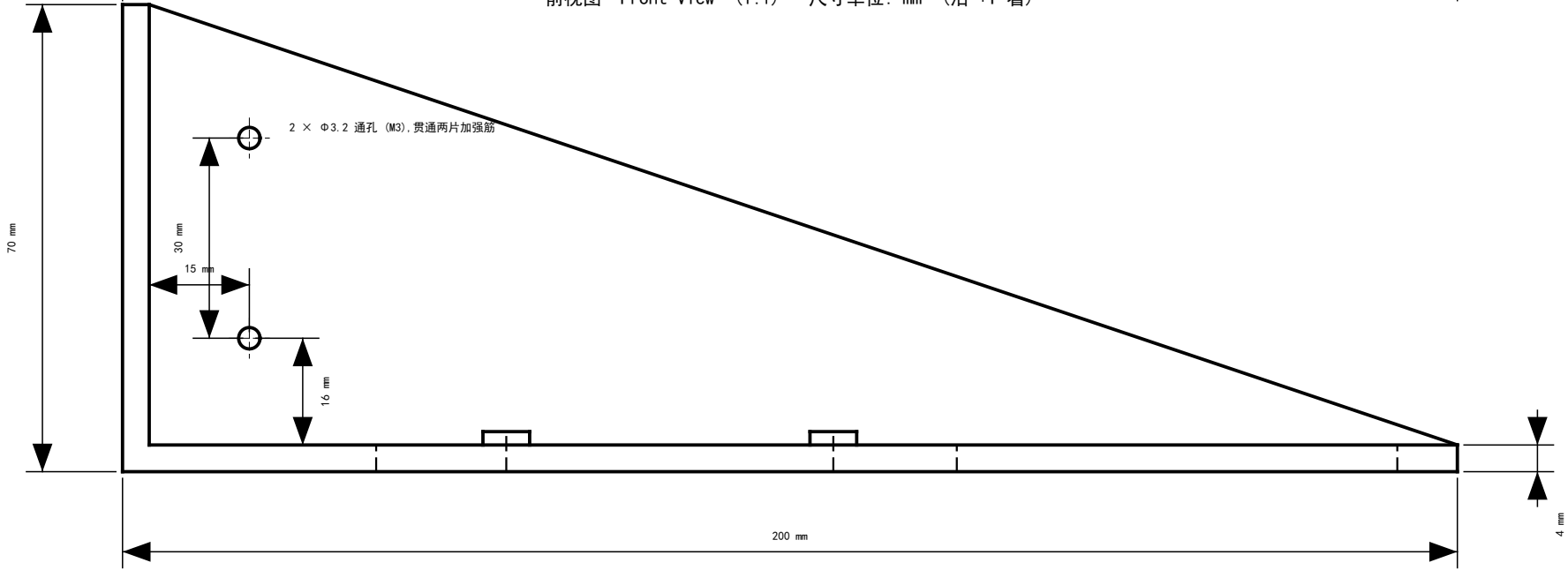
前视图 Front View (1:1) 尺寸单位: mm (沿 +Y 看)
