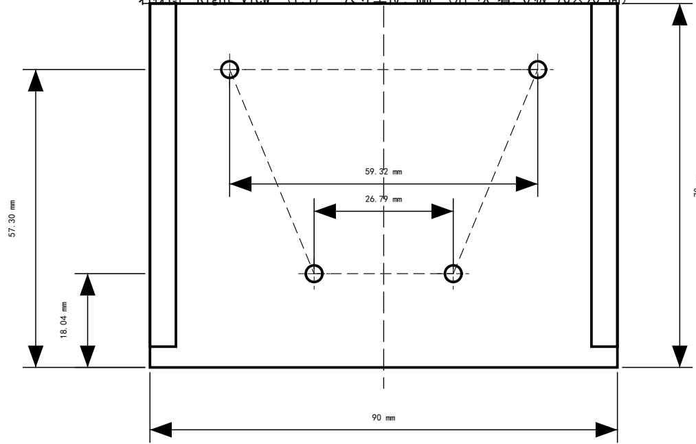
右视图 Right View (1:1) 尺寸单位: mm (沿 +X 看 立板 70×90 面)
