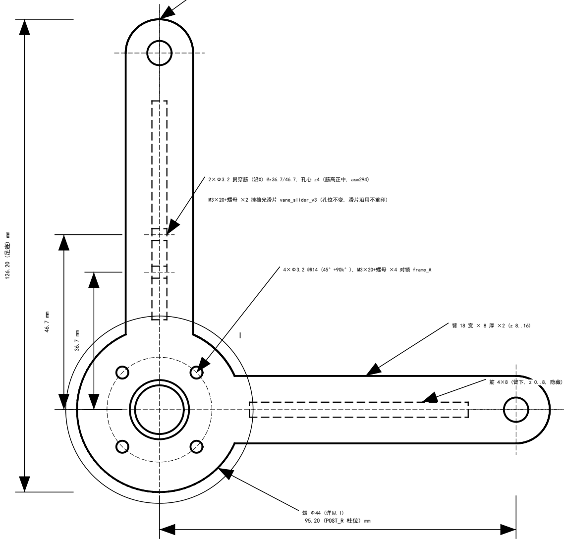
俯视图 (X-Y, 1:1)
