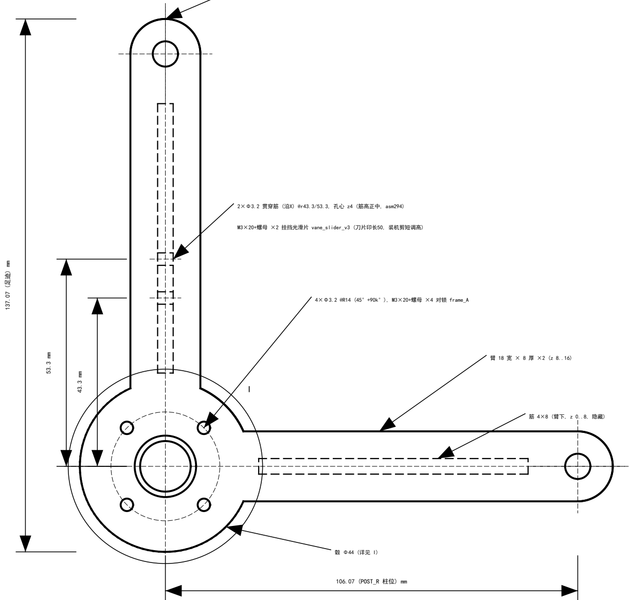
俯视图 (X-Y, 1:1)
