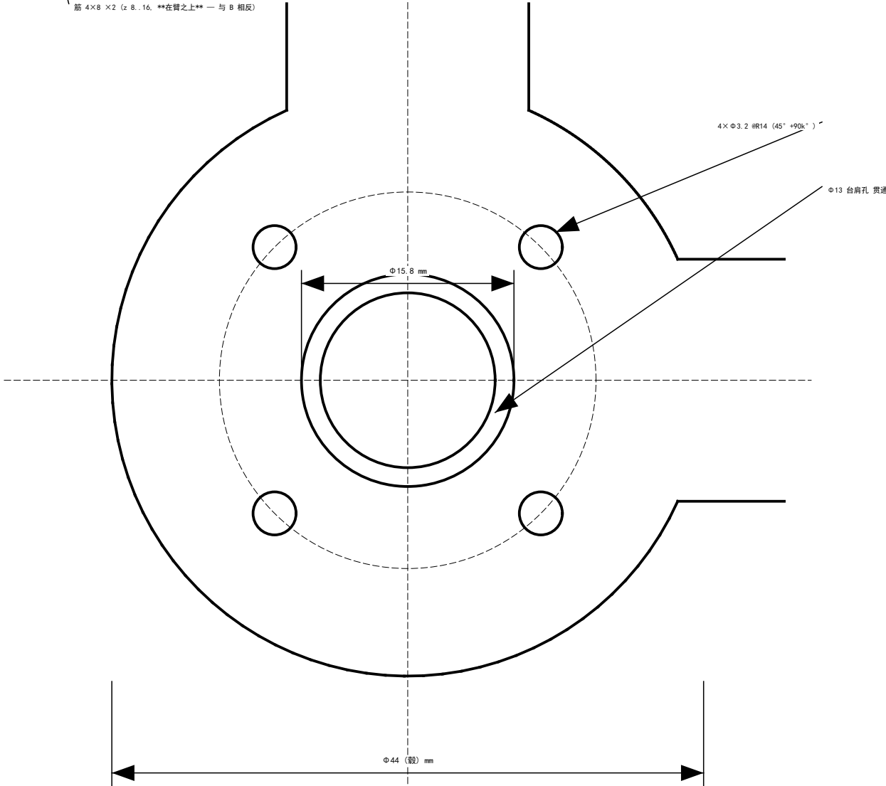
局部放大 I（毂 俯视, 2.5:1）
