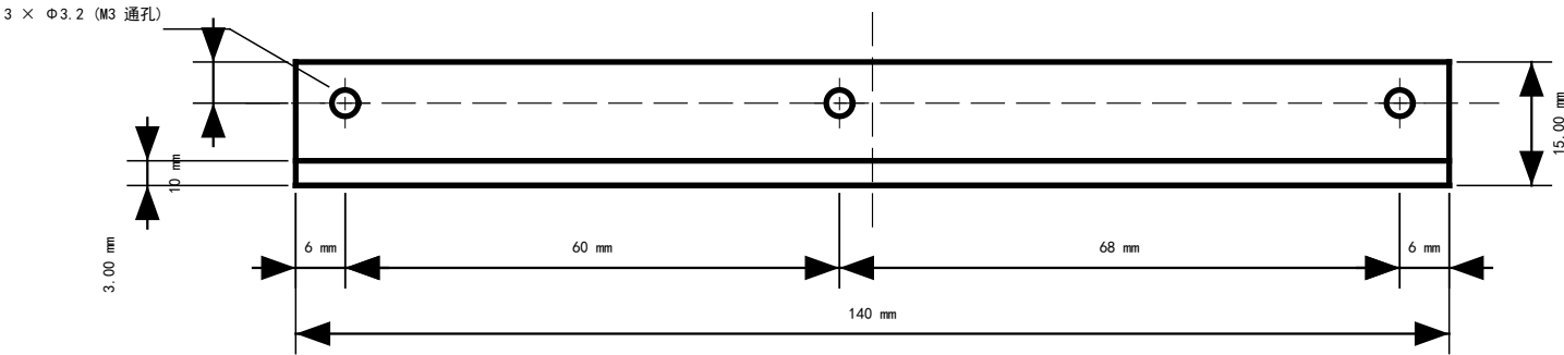
俯视图 Top View (1:1) 尺寸单位: mm
