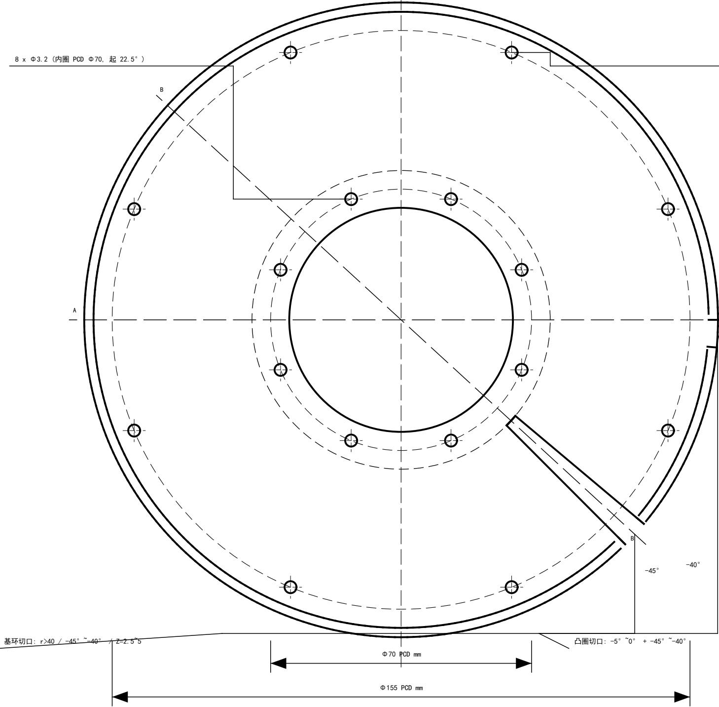
俯视图 Top View (1:1) 尺寸单位: mm
