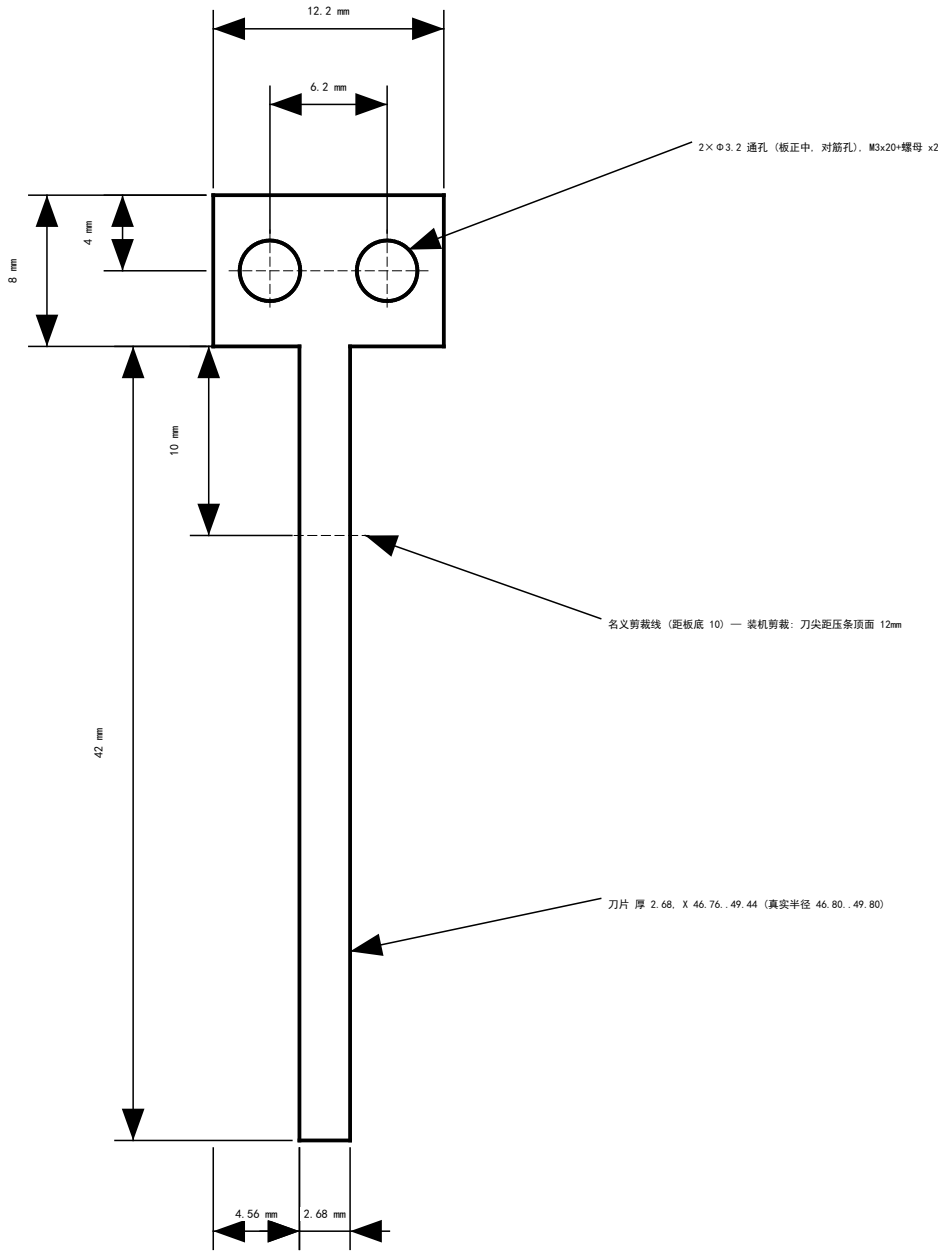
主视图 (2.5:1)
