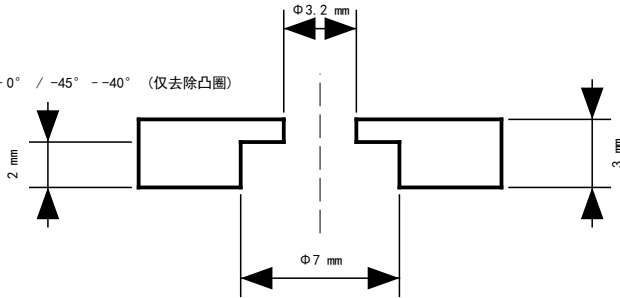
详图 B Detail B (3:1) 尺寸单位: mm
