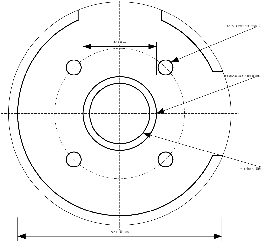
局部放大 I (毂, 俯视 2.5:1)
