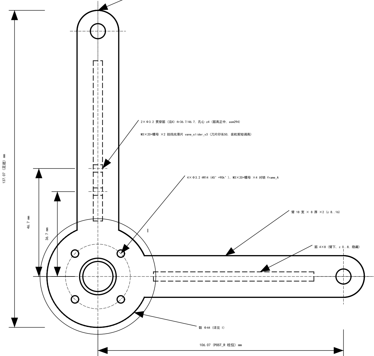
俯视图 (X-Y, 1:1)
