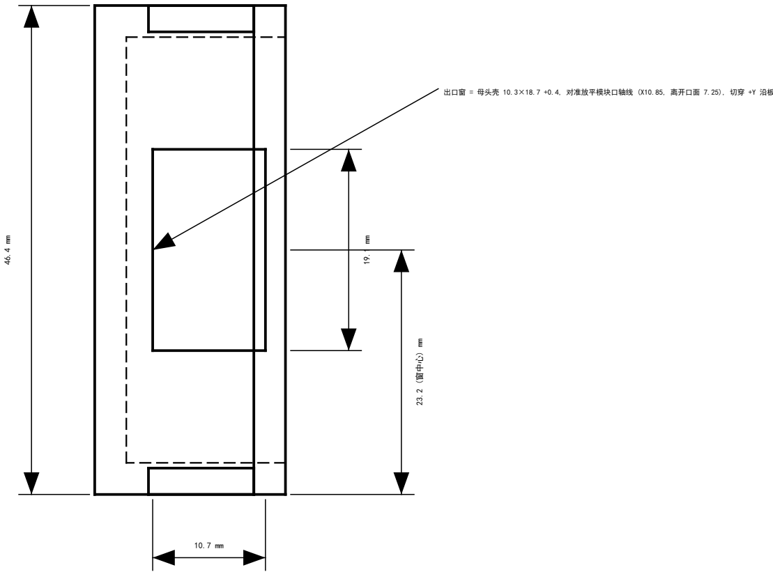
正视图 (从 +Y 端看, 2:1) — 出口窗
