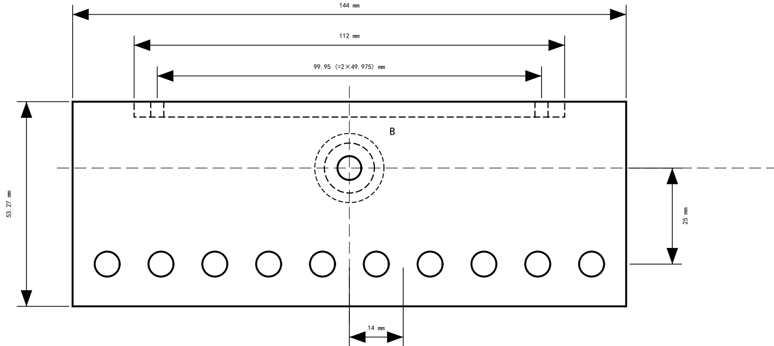
俯视 (1:1) (沿 -Z 看顶面) 尺寸单位: mm
