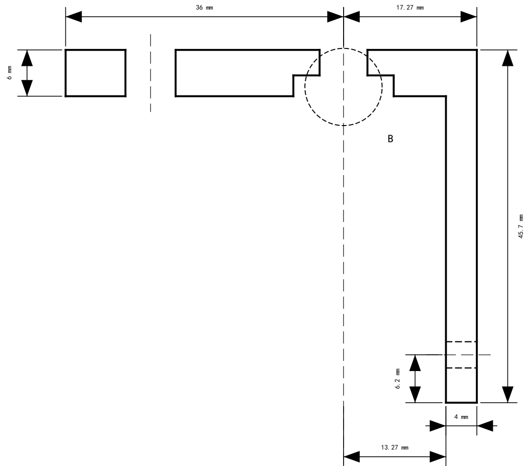
侧视剖面 (2:1) (沿 +Y 看, 剖切面 Y=0 ) — L型, 腿在+X端
