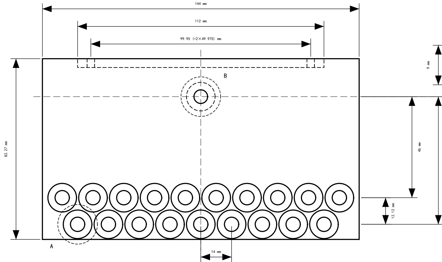
俯视 (1:1) (沿 -Z 看顶面) 尺寸单位: mm
