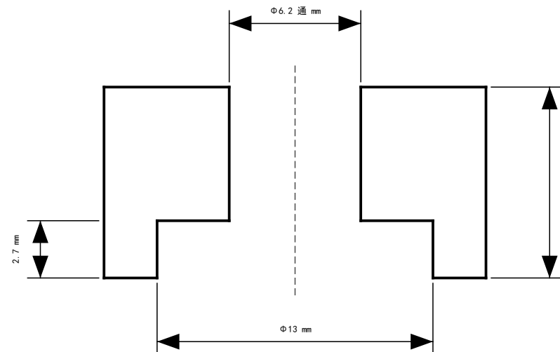
详图 B (4:1) 轴孔头窝 — 底面进 (方向与A相反)
