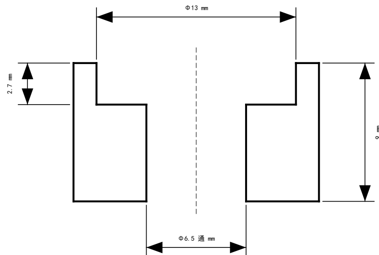
详图 A (4:1) 配重沉孔 — 顶面进
