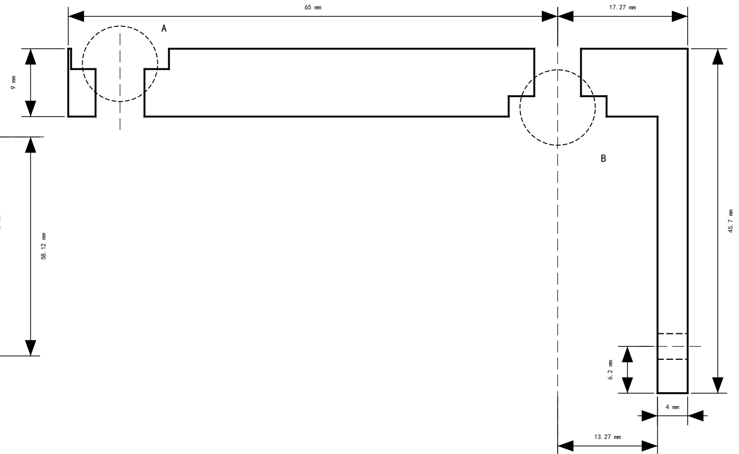
侧视剖面 (2:1) (沿 +Y 看, 剖切面 Y=0 ) — L型, 腿在+X端
