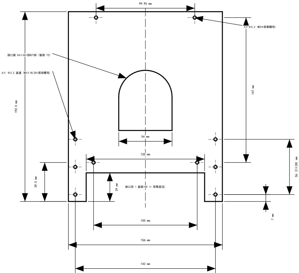
主视图（前面/贴屏面，1:2）
