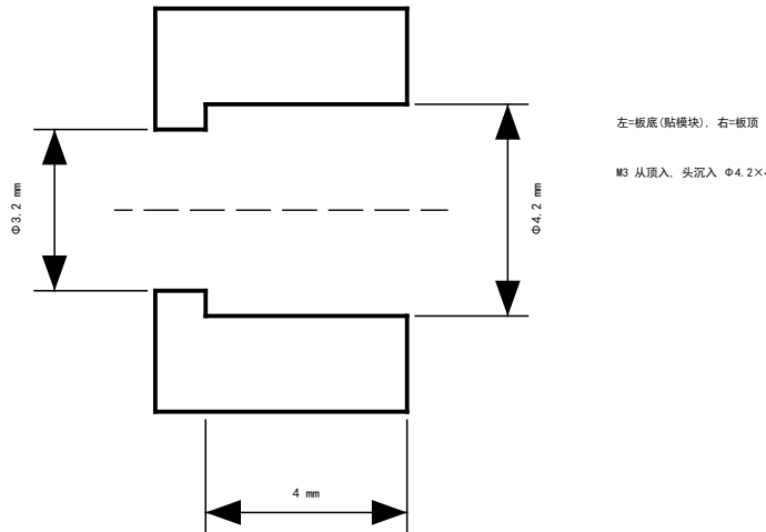
详图 A (6:1) — 模块孔 Φ4.2 顶沉
