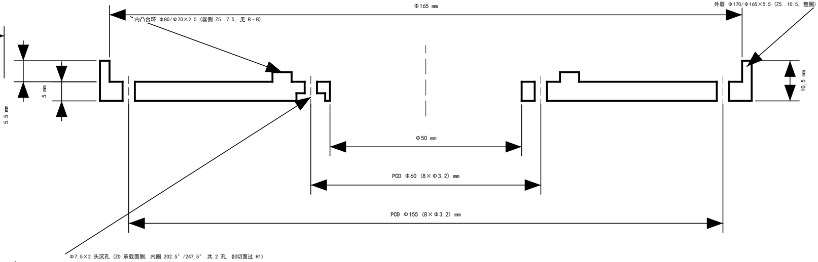
剖面 B-B (2:1) — 沿 -42.5^\circ 半径半剖 尺寸单位: mm
