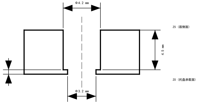
详图 C (4:1) 尺寸单位: mm
