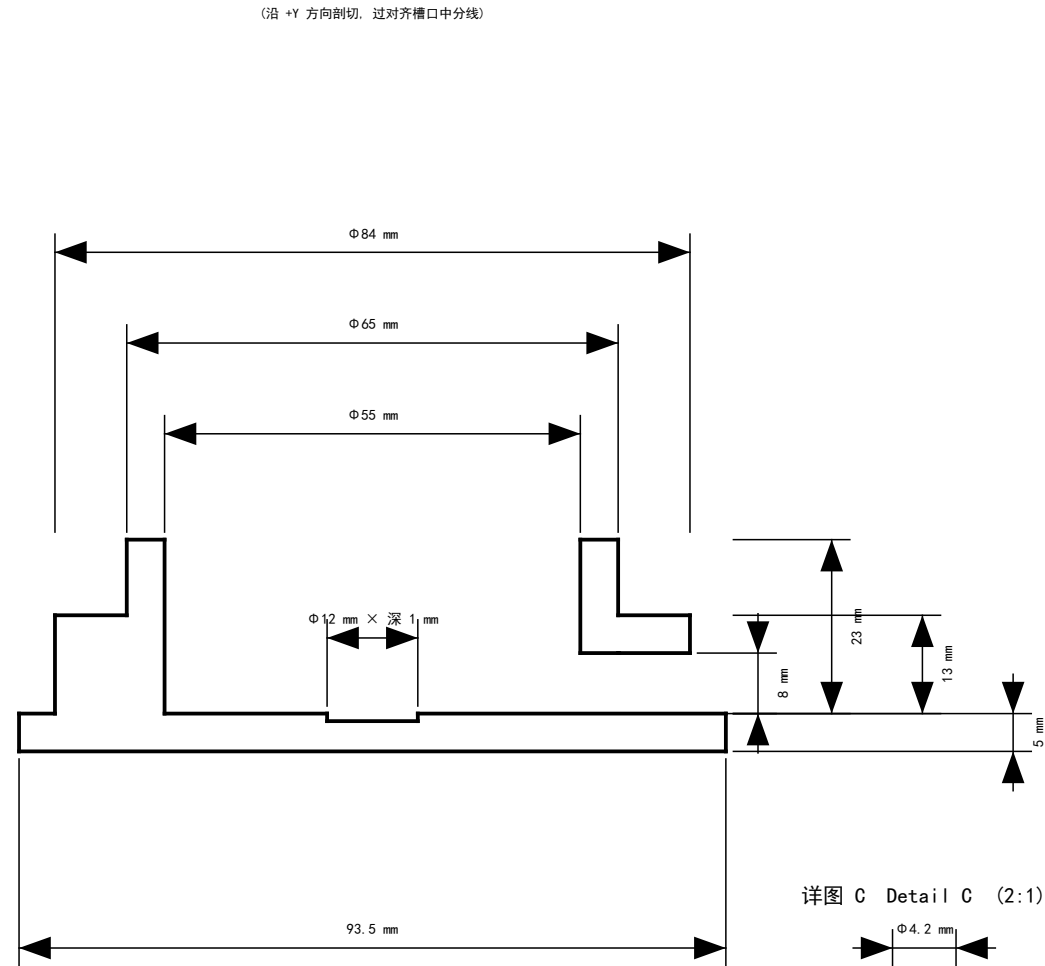
剖视图 Section A-A (1:1) 尺寸单位: mm
