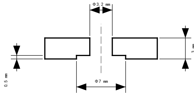
详图 B Detail B (3:1) 内圈孔 (PCD \Phi 72.5 ) 尺寸单位: mm
