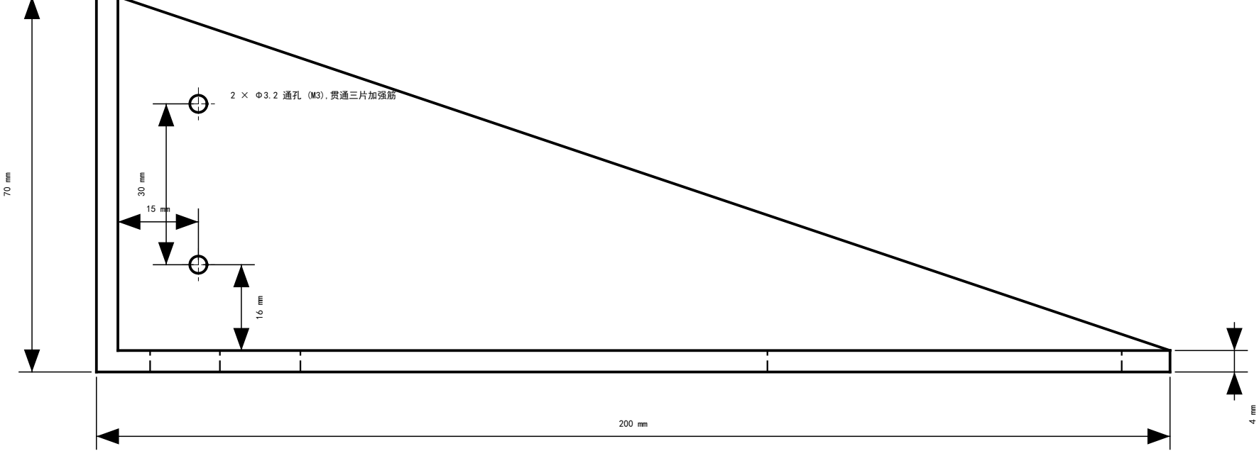
前视图 Front View (1:1) 尺寸单位: mm (沿 +Y 看)
