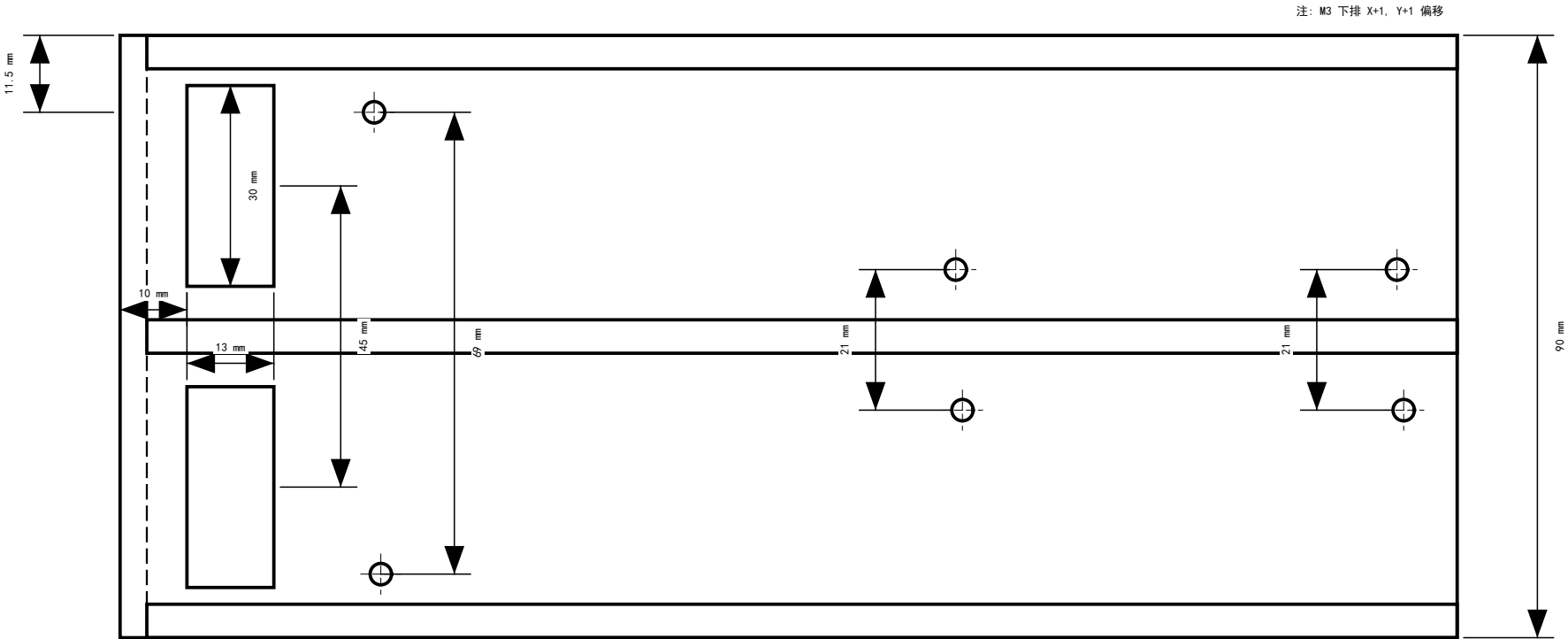
俯视图 Top View (1:1) 尺寸单位: mm (沿 -Z 看)
