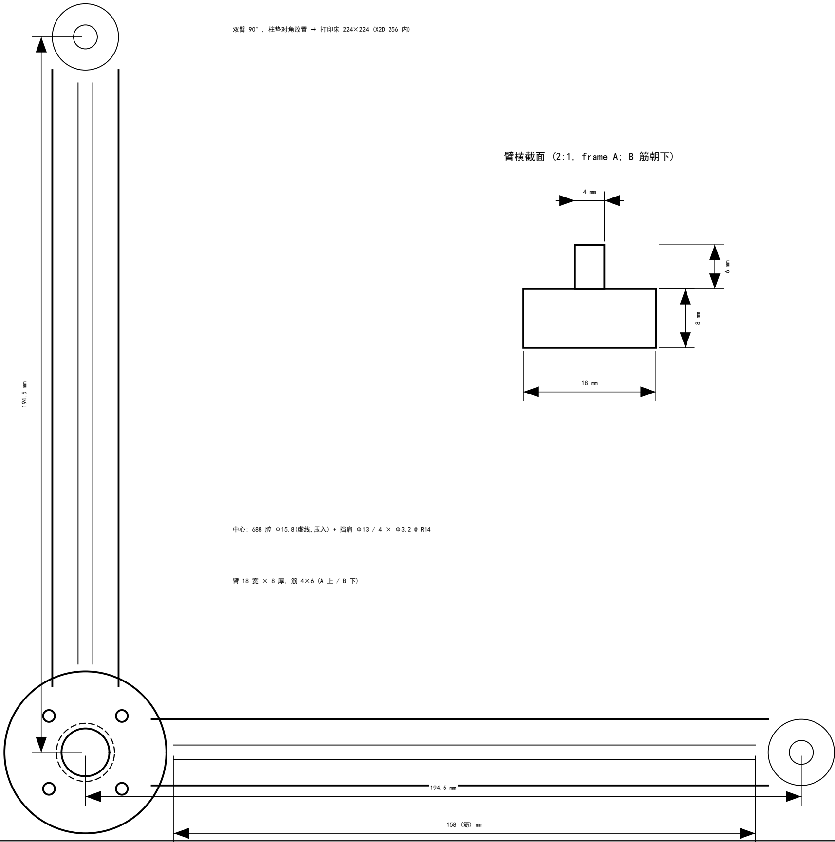
frame_A 俯视（1:1） 尺寸单位：mm
